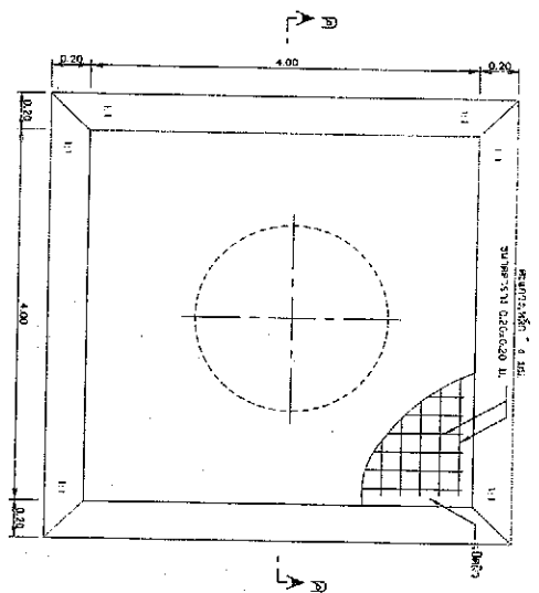
แบบพื้นคอกคอนกรีตเสริมเหล็ก
