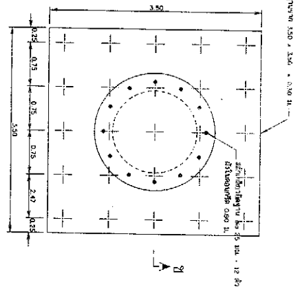
แบบฐานฐานหลักสูง (แบบฐานหลัก)
