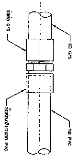
2. แผนการวางท่อ G/S กับท่อ PVC
