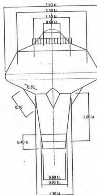
แบบขยายแมนโซลบนหัวฉีดสูง มาตรฐาน 1 : 50
