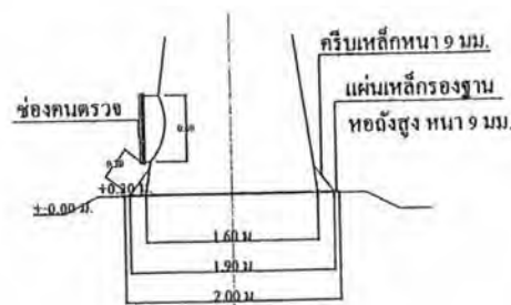
แบบขยายแมนโซลล่างหัวฉีดสูง มาตรฐาน 1 : 50
