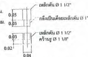
แบบขยายบานพับรั้วเหล็ก
