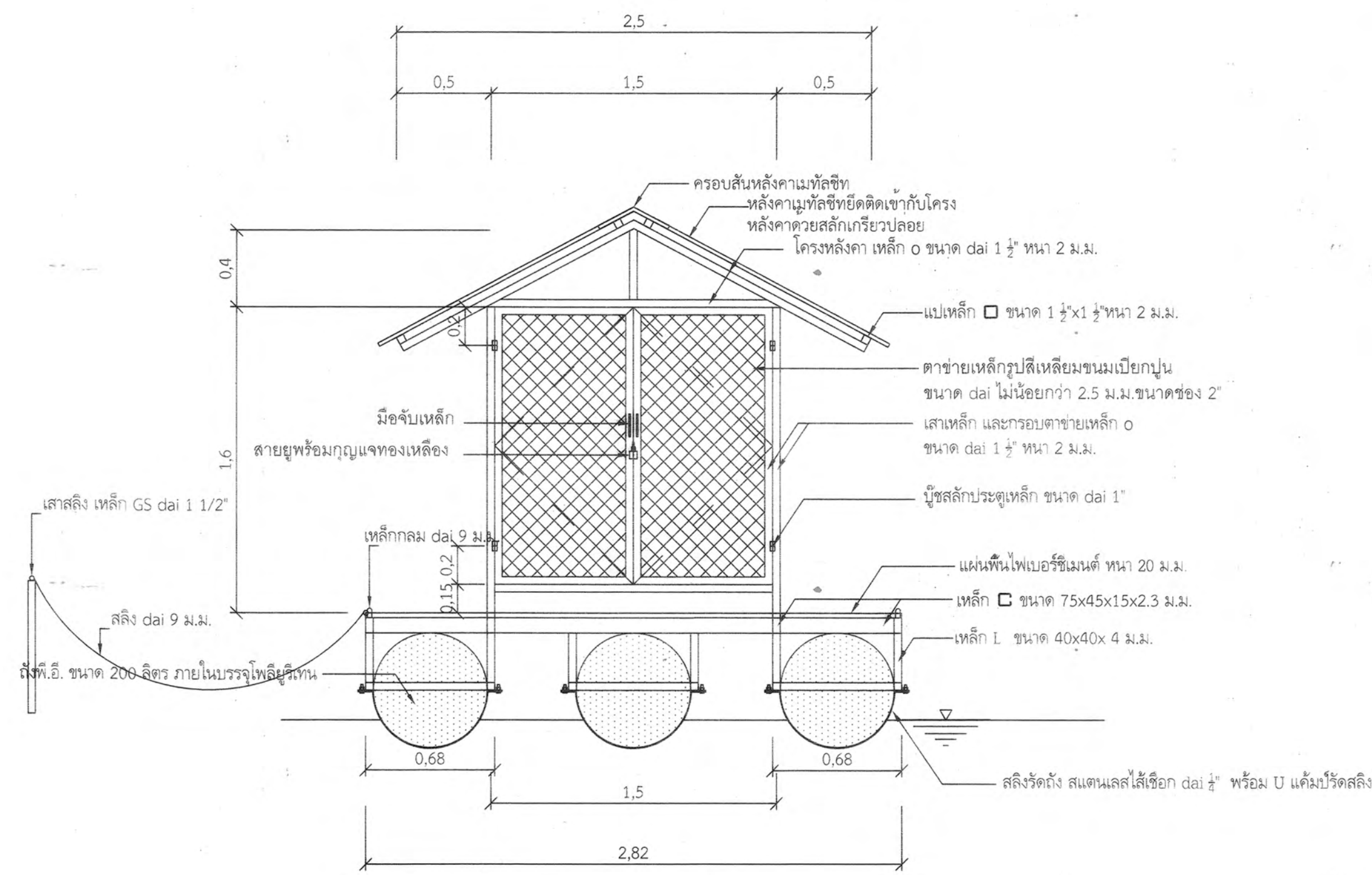
รูปด้านหน้า 1:25
