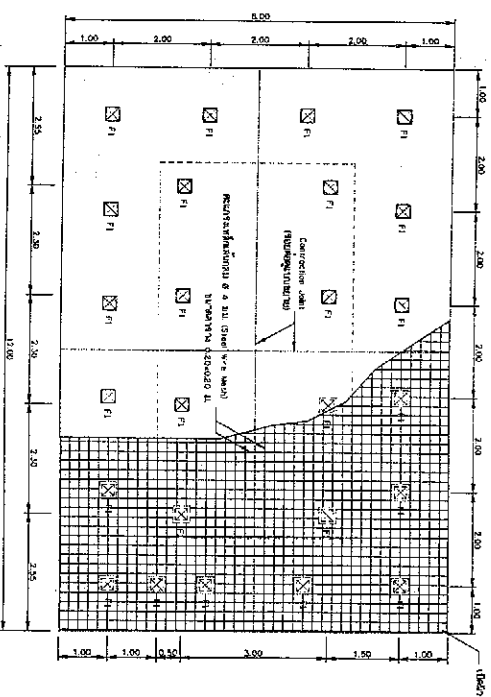
รูปขยายพื้นคอนกรีต
