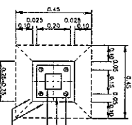
รูปตัด ก-ก
