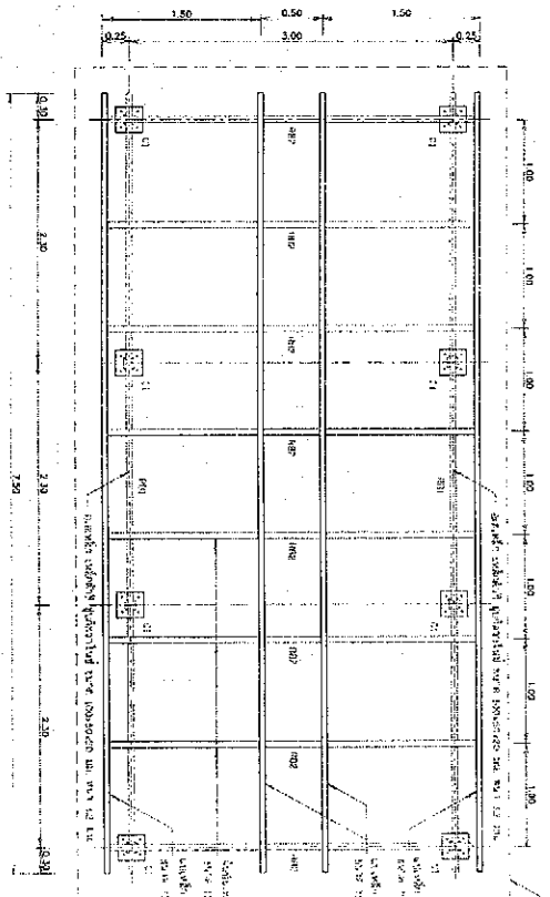
แปลนฐานรากและโครงสร้างเสถียร
