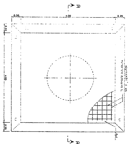
แปลนเสาเข็มกริดเสริมเหล็ก
