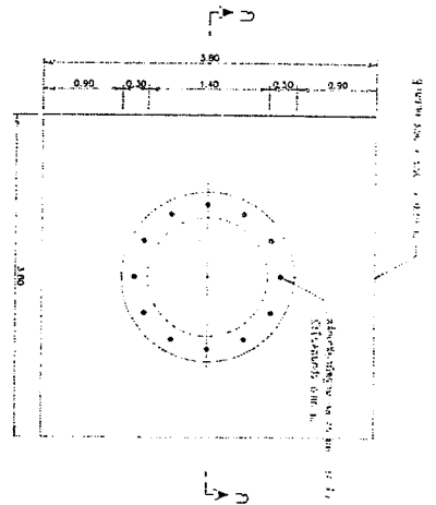
แปลน ฐานรากหล่อสูง (แบบฐานกลม)
