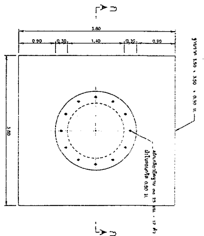
แบบฐาน ฐานรากหอยต่งสูง (แบบฐานแผ่) โน้ตตามตาราง
