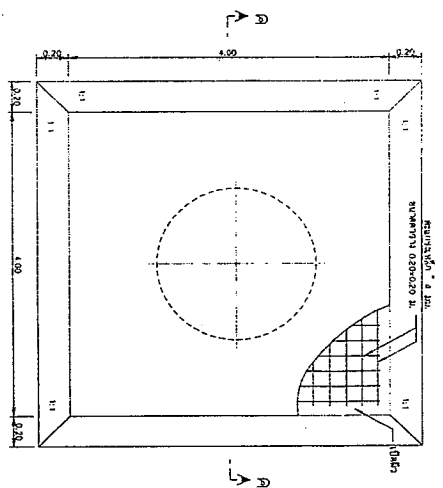
แบบฐาน ฐานคานยก (แบบคานยก) โน้ตตามตาราง
