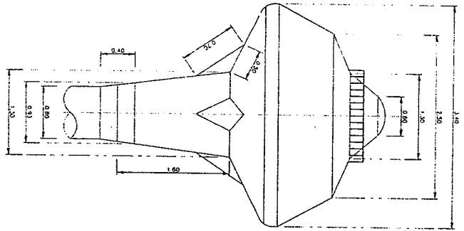
แบบขยายผนัง โคลนบนหลังคา
