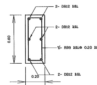
แบบขยาย A
