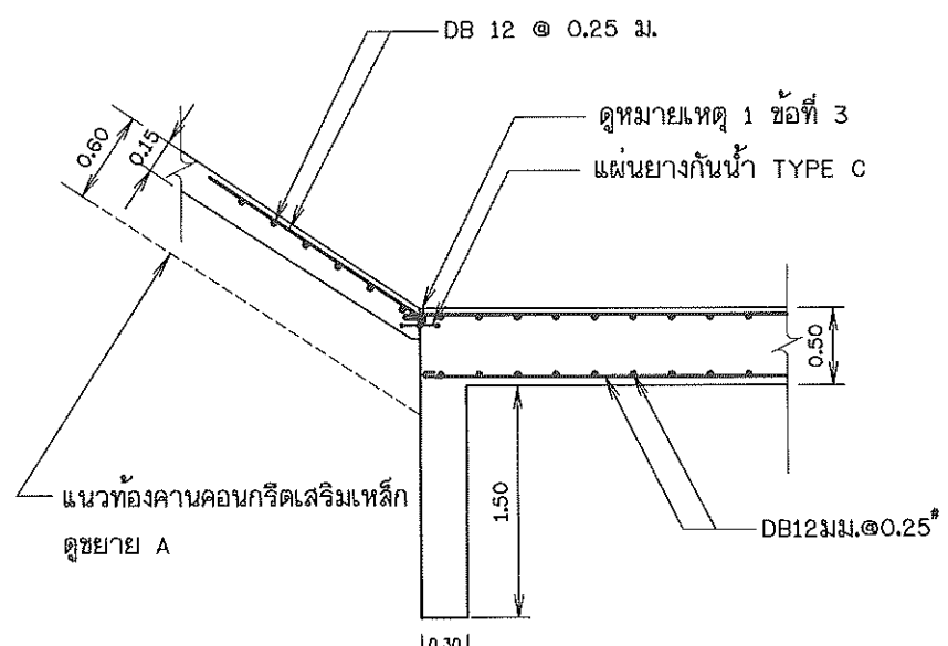
รูปตัด B
