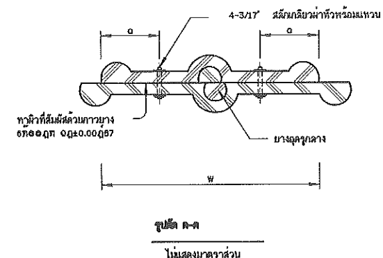
การต่อพาดทับกันไม่ทำมุมฉาก ไม่แสดงขนาดส่วน
