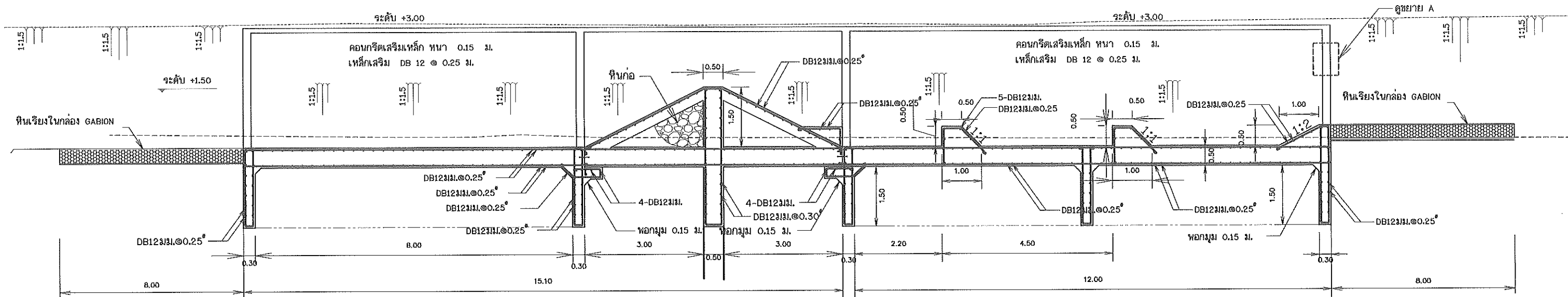
รูปตัด แสดงการเสริมเหล็ก
