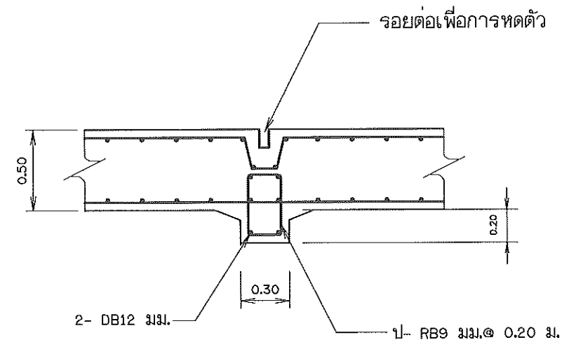
แบบขยาย C
