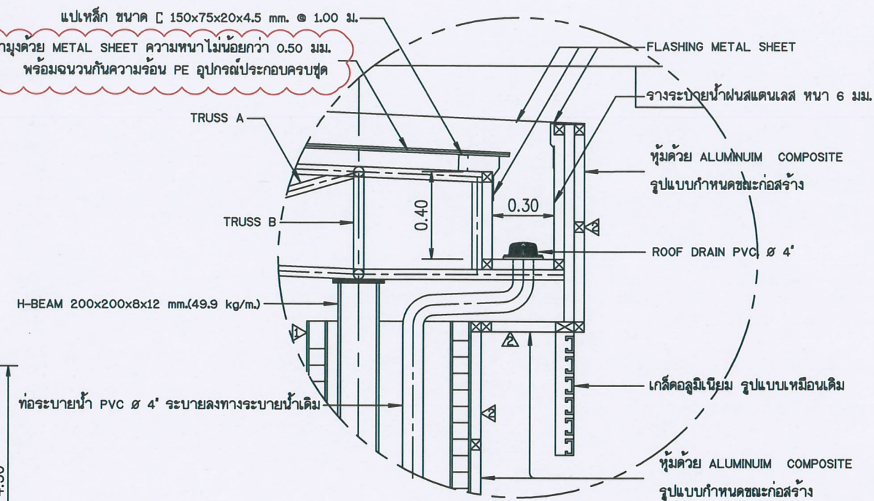
ขยาย รางระบายน้ำ มาตราส่วน 1:25
