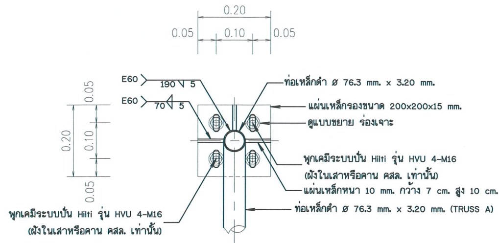
ขยาย 1 มาตราส่วน 1:10
