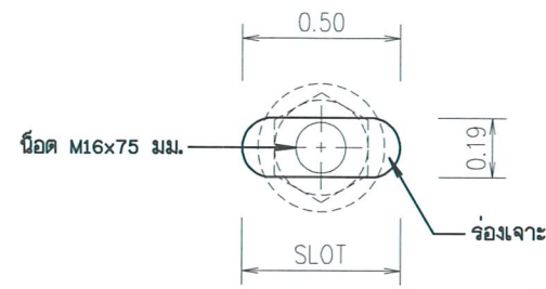
ขยาย ร่องเจาะ มาตราส่วน 1:2.5
