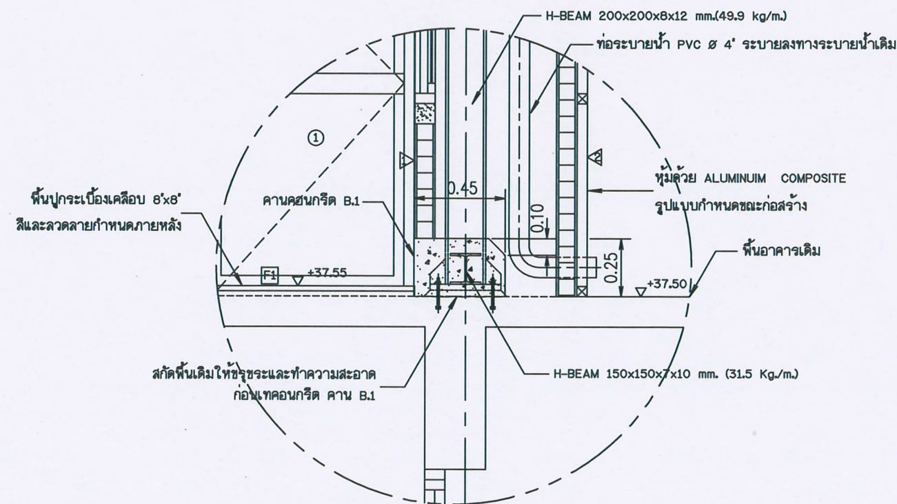
ขยาย คาน B.1 มาตราส่วน 1:25
