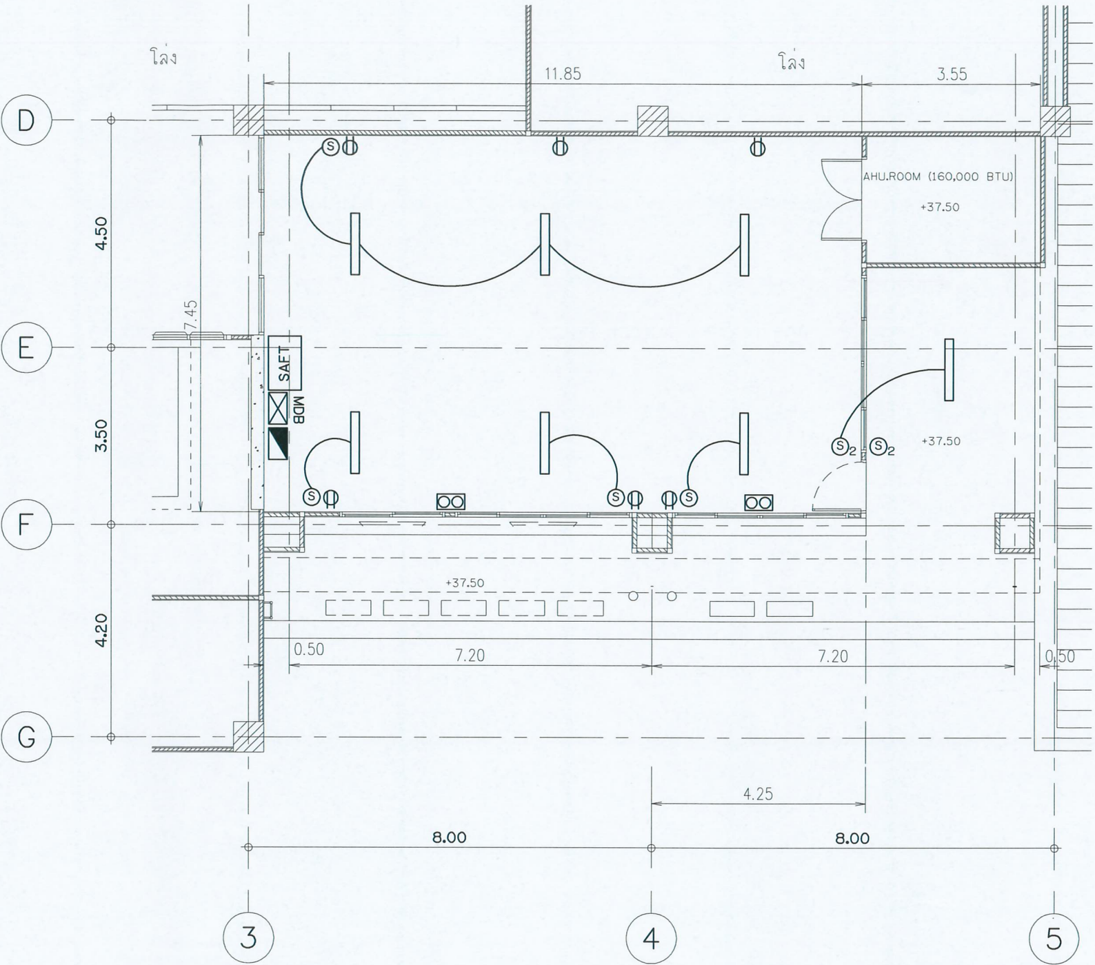
แปลนไฟฟ้าและระบบปรับอากาศ มาตราส่วน 1:100
