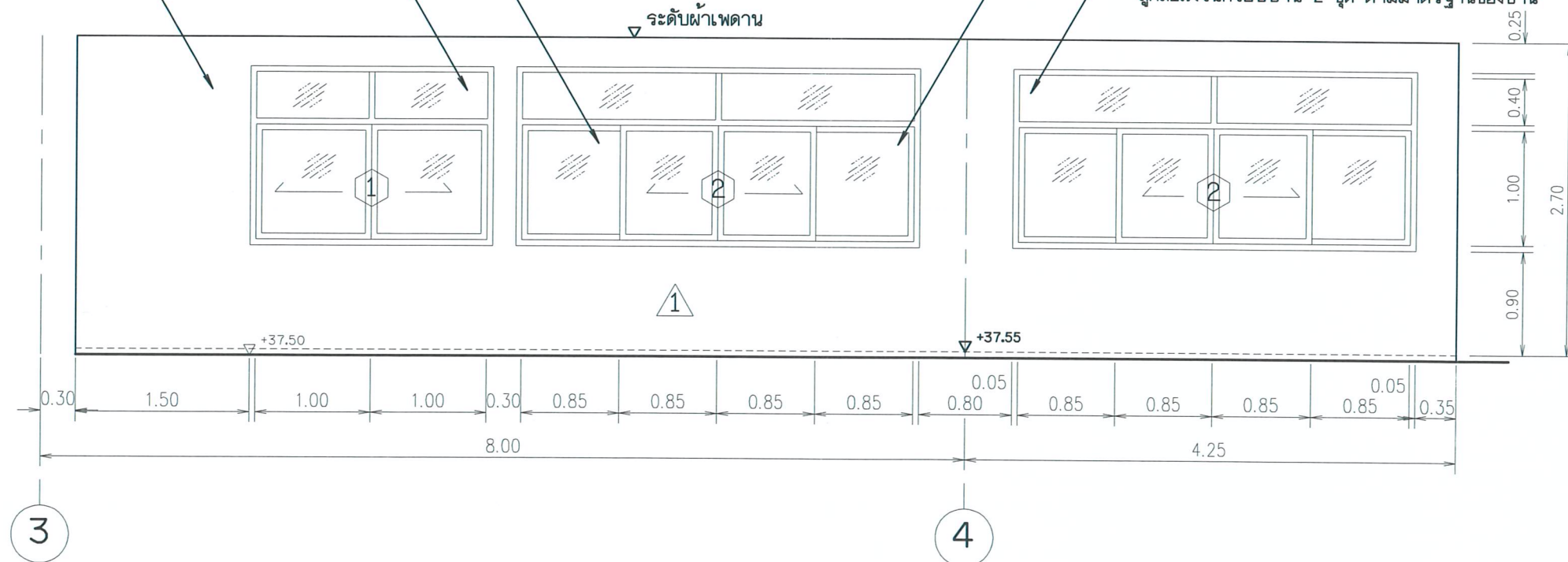
รูปด้านผนัง B
