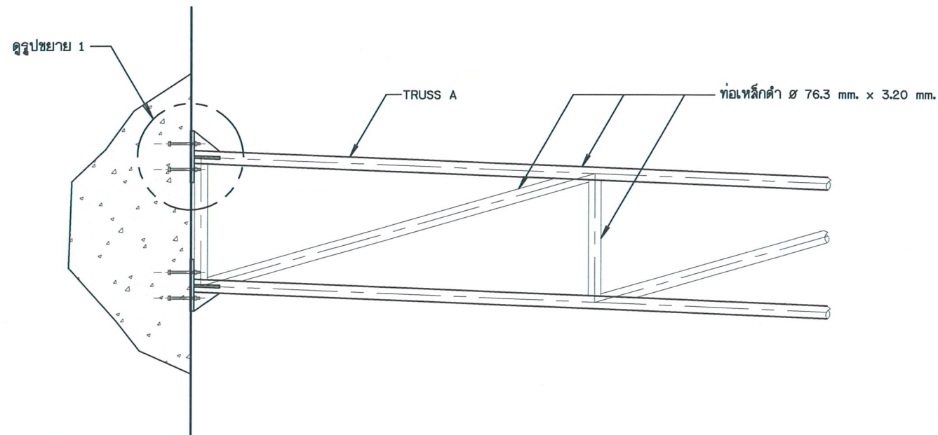
ขยาย การติดตั้ง TRUSS (A) กับผนัง มาตราส่วน 1:20
