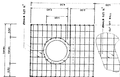
รูปดำเนิน. ด้านนอก(แสดงการเสริมเหล็ก)
