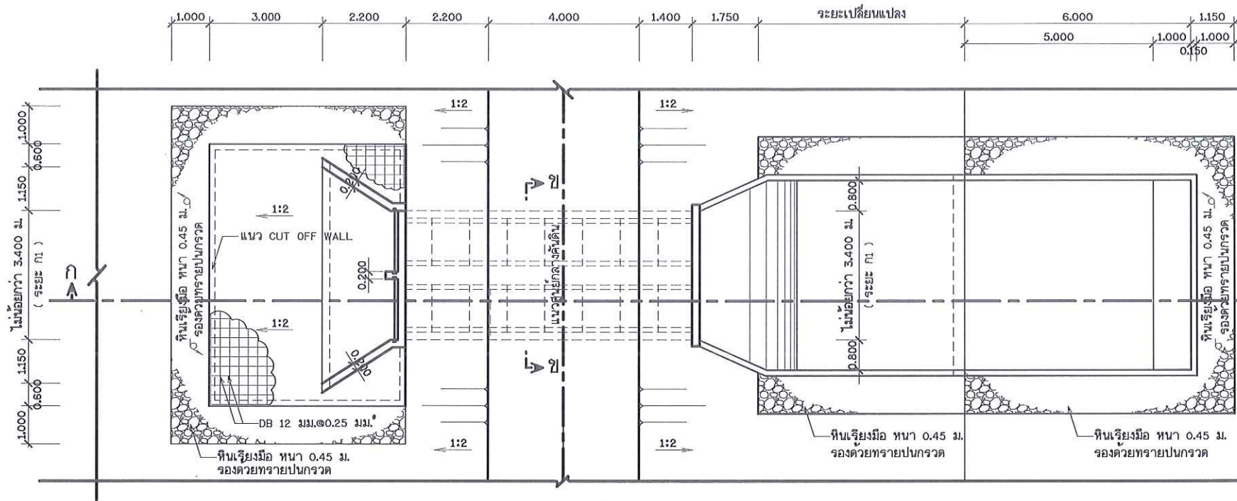
แปลนอาคารระบายน้ำ 2-Ø 1.00 ม. มาตราส่วน 1:100
