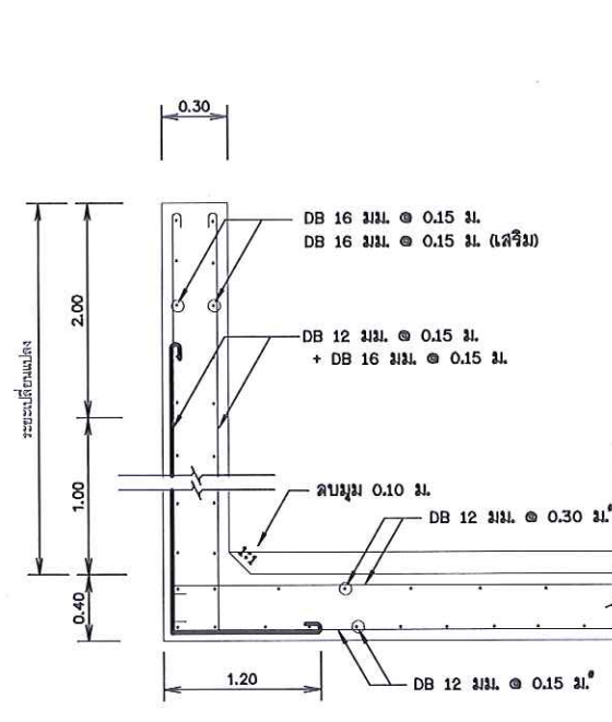
รูปตัด "ค" มาตราส่วน 1:20
