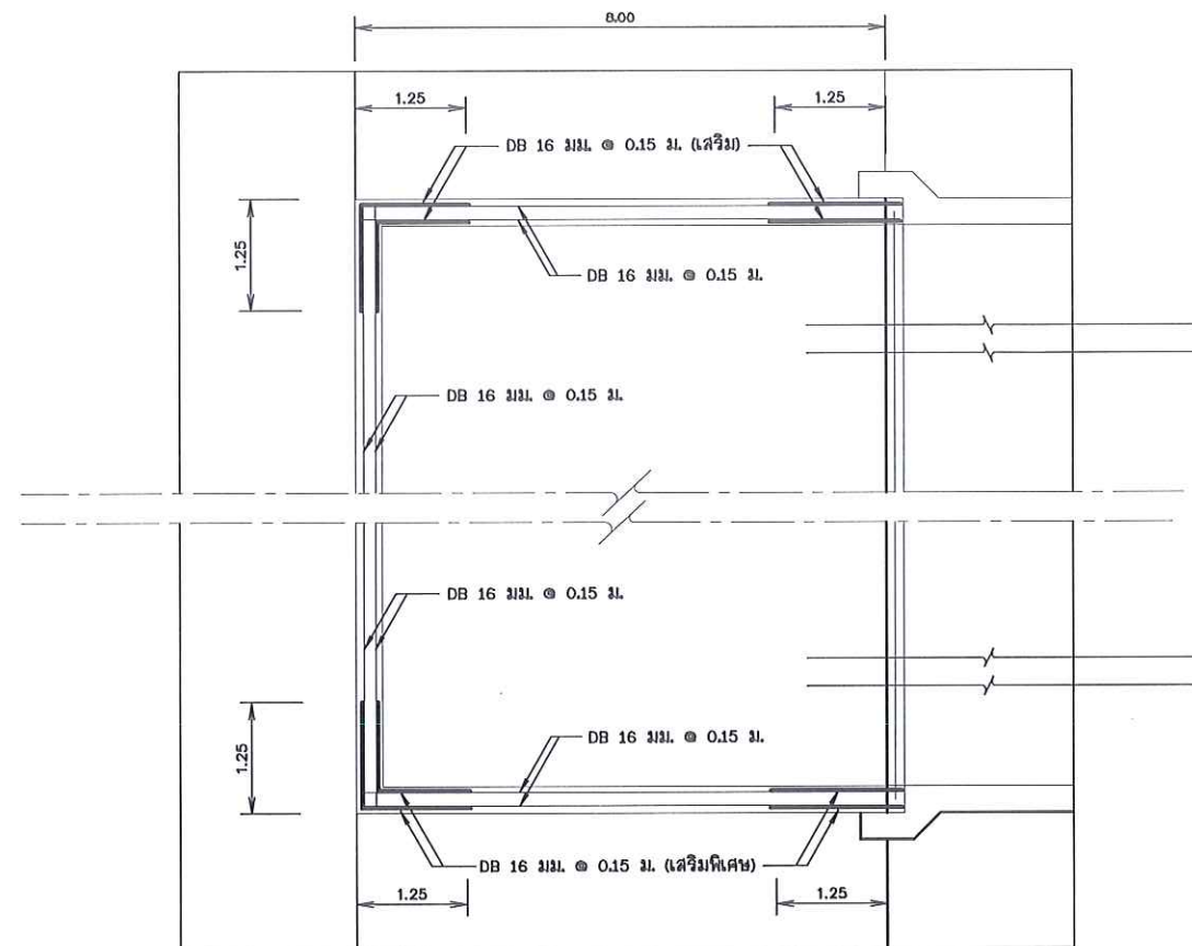
แปลนขยายเหล็กกำแพง มาตราส่วน 1:25
