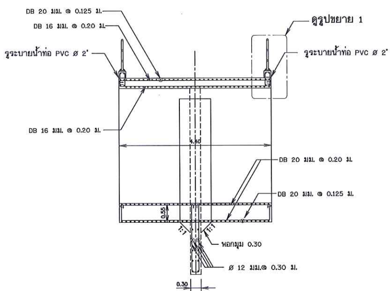
รูปตัดตามยาวท่อเหลี่ยม คสล.
