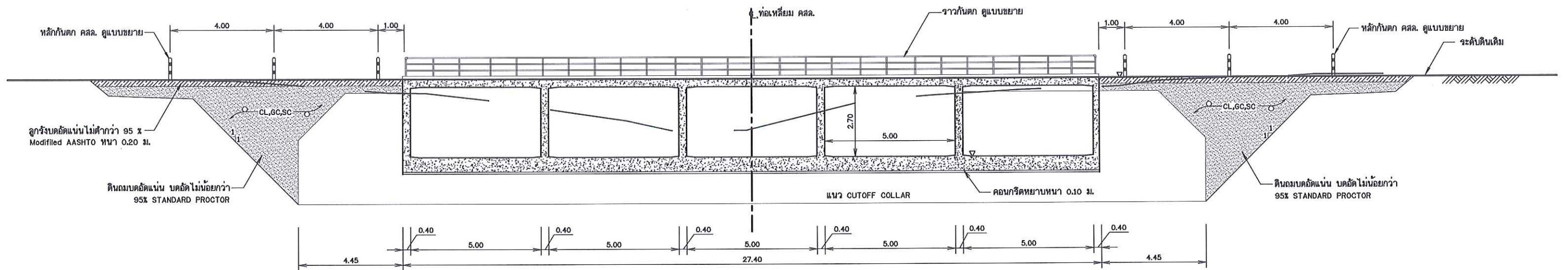
รูปตัดตามขวางแนว ข - ข
