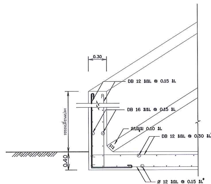
แปลนขยายเหล็กกำแพง มาตราส่วน 1:25
