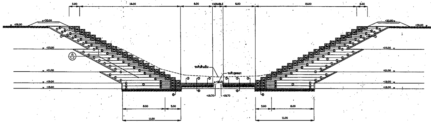
ตัวอย่างรูปตัดทั่วไปแสดงการขุดลอก และการป้องกันการกัดเซาะหินเรียงในกล่อง GABION
