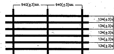
รูปแบบตัวอย่างวัสดุเสริมกำลังดิน ชนิดที่ 1 กำลังรับแรงดึงสูงสุดไม่น้อยกว่า 175 KN/m.
