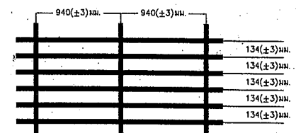
รูปแบบตัวอย่างวัสดุเสริมกำลังดิน ชนิดที่ 2 กำลังรับแรงดึงสูงสุดไม่น้อยกว่า 125 KN/m.
