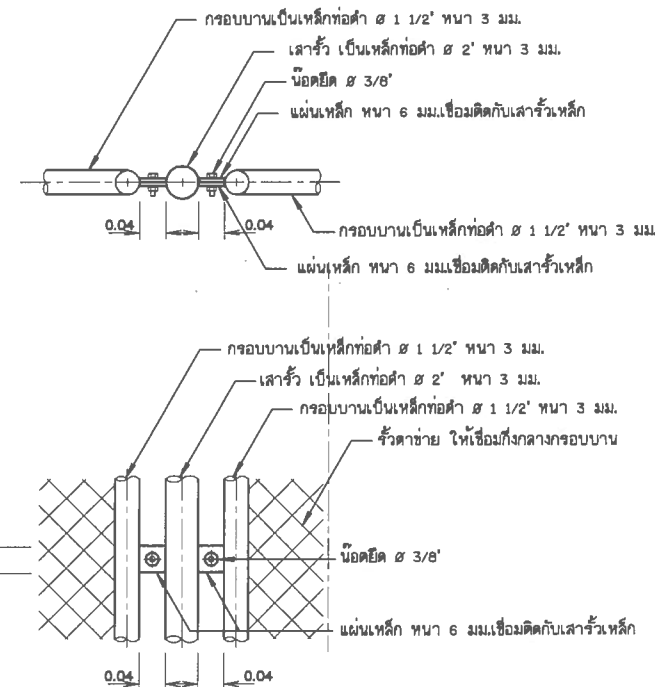
แบบขยายรายละเอียดแสดงการยึดระหว่างหัวกับเสา ไม่แสดงขนาดบางส่วน
