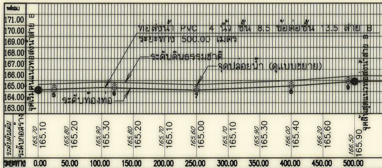
รูปตัดตามยาวท่อส่งน้ำ สาย B
