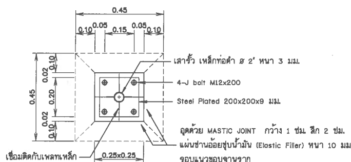
รูปตัด ข-ข ไม่แสดงขนาดบางส่วน
