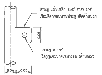
แบบขยายสายยู ไม่แสดงขนาดบางส่วน
