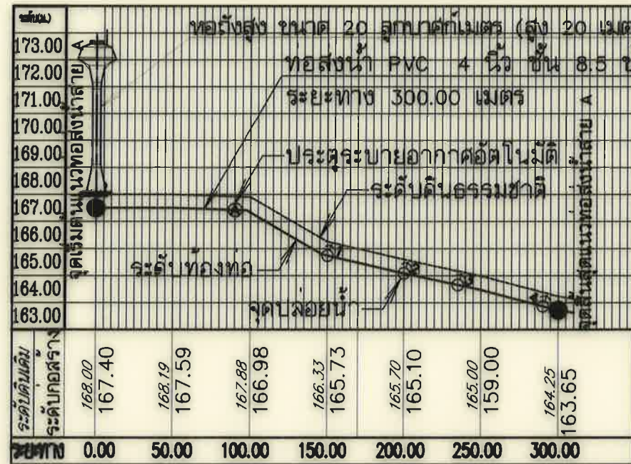
รูปตัดตามยาวท่อส่งน้ำ สาย A
