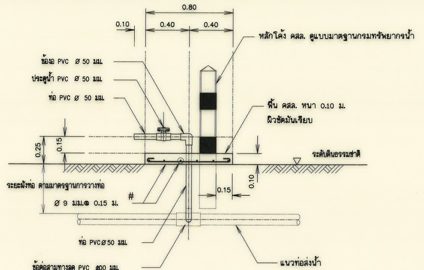
รูปตัด ก - ก แสดงการติดตั้งประตูจุดปล่อยน้ำ
