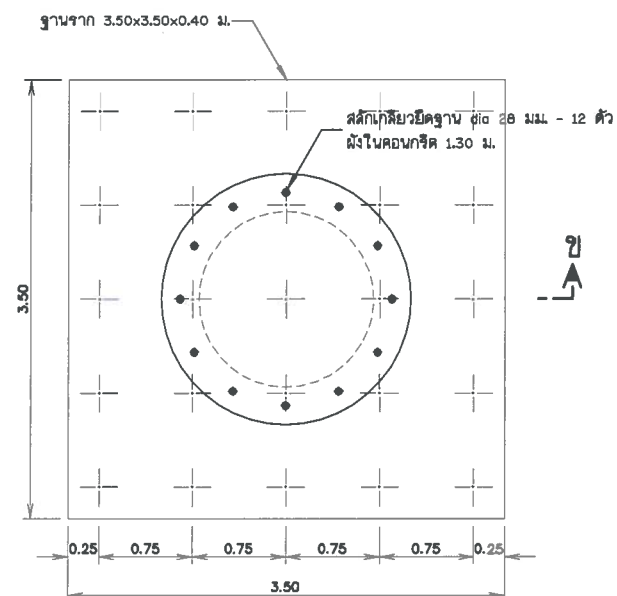
แปลน ฐานรากหอลังสูง (แบบเสาเข็ม)
