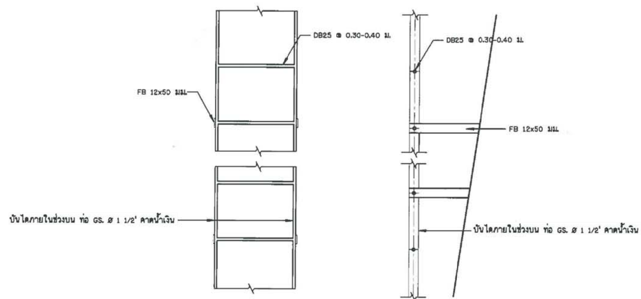
แบบขยายบันได ภายในหอดึงสูง ไม่แสดงมาตราส่วน
