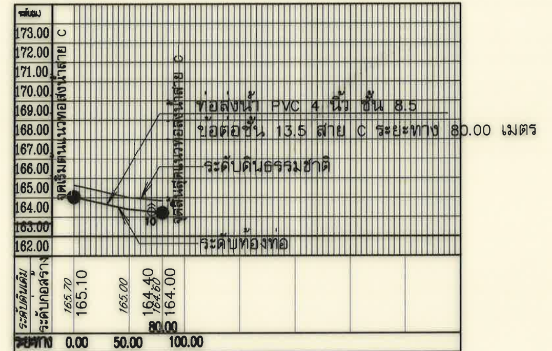
รูปตัดตามยาวท่อส่งน้ำ สาย C
