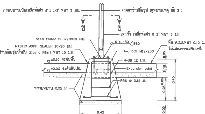
รูปขยายฐานรากโครงสร้างรับแผง F1 (ต่อม่อ คสล. ห่อสำหรับรูปพร้อมติดตั้ง) ไม่แสดงขนาดบางส่วน
