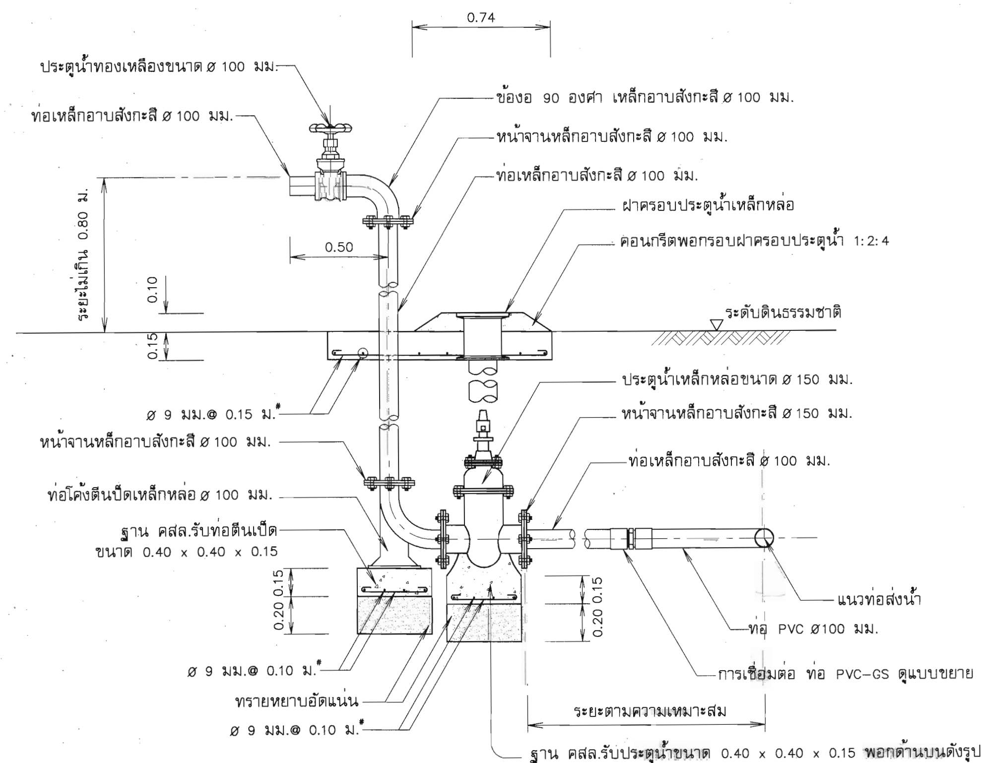
รูปตัด ก - ก อาคารระบายตะกอน
