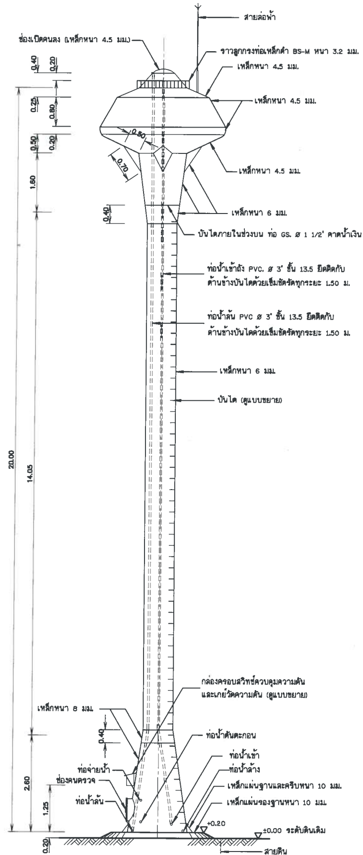
รูปด้านข้างของถังสูง แบบถังเหล็กรูปทรงแปดเหลี่ยม ไม่แสดงมาตราส่วน
