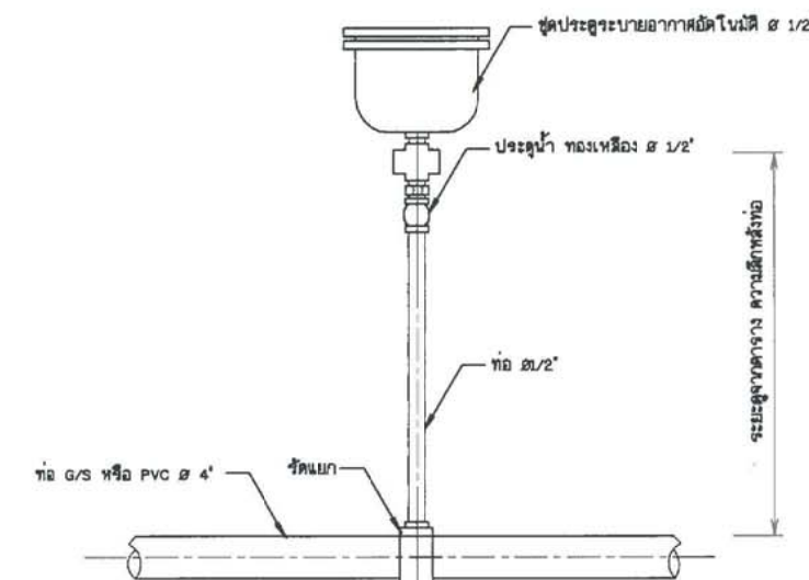
12. การติดตั้งประจุสารอากาศอัดไนโตรเจน ไม่แสดงมาตราส่วน
