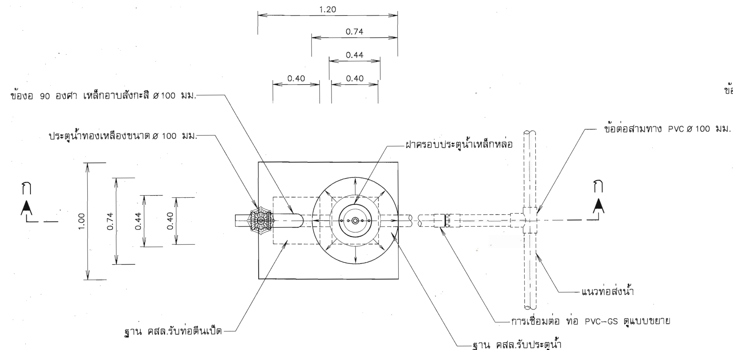
แปลนอาคารระบายตะกอน
