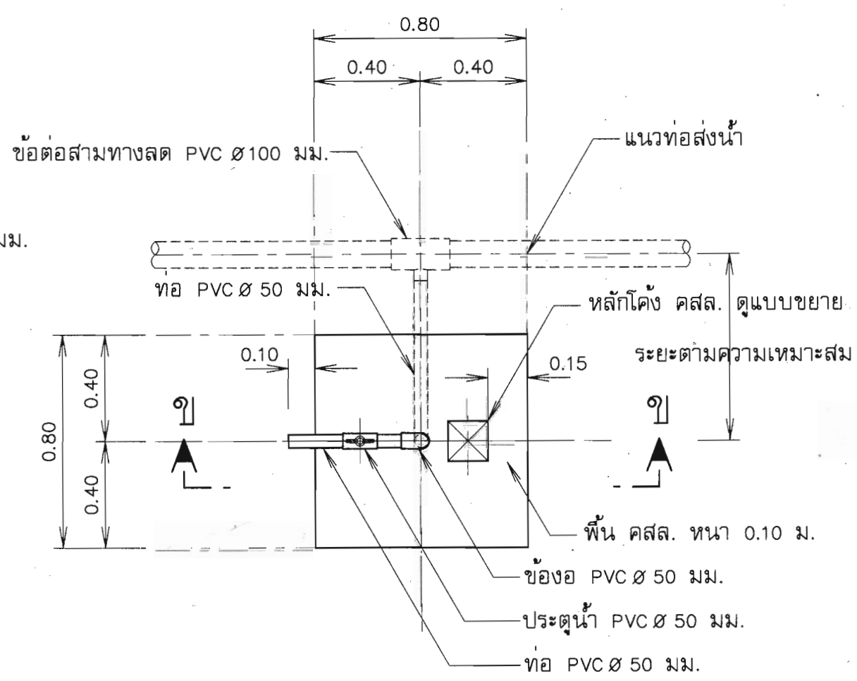
แปลนอาคารจุดปล่อยน้ำ
