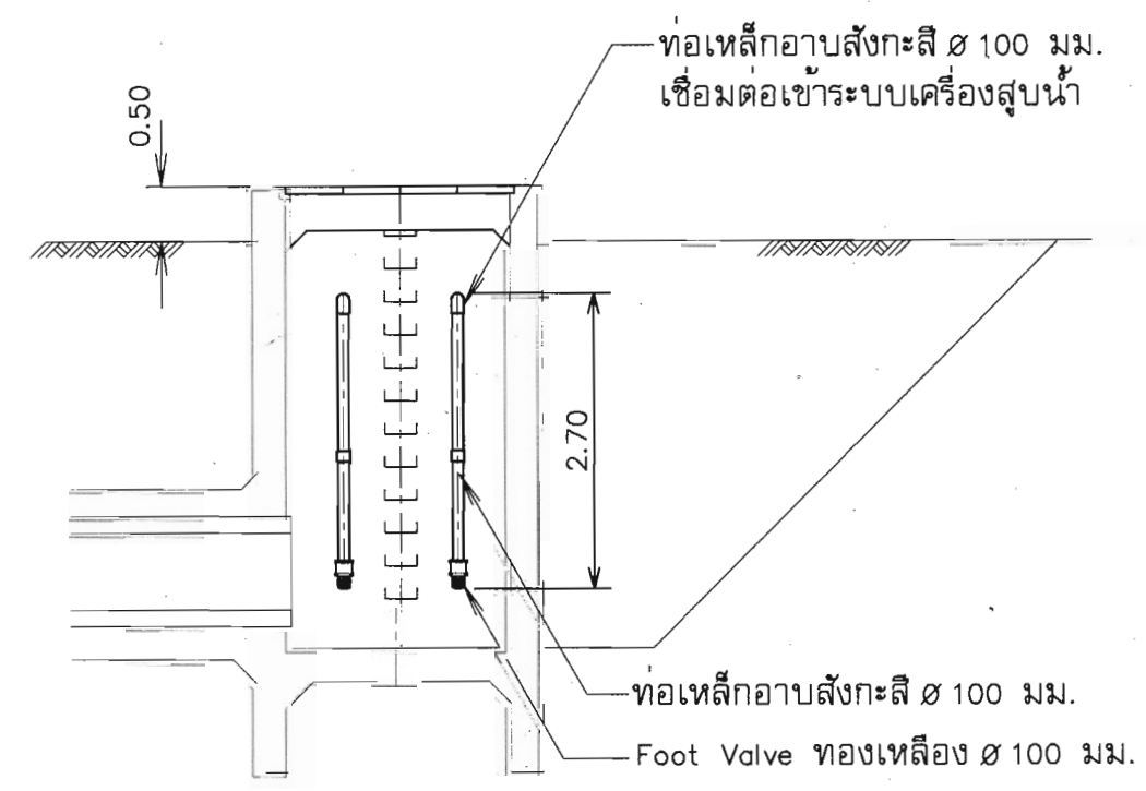
แบบขยายการเดินท่อแหล่งน้ำดิบจากอาคารบังคับน้ำเดิม
