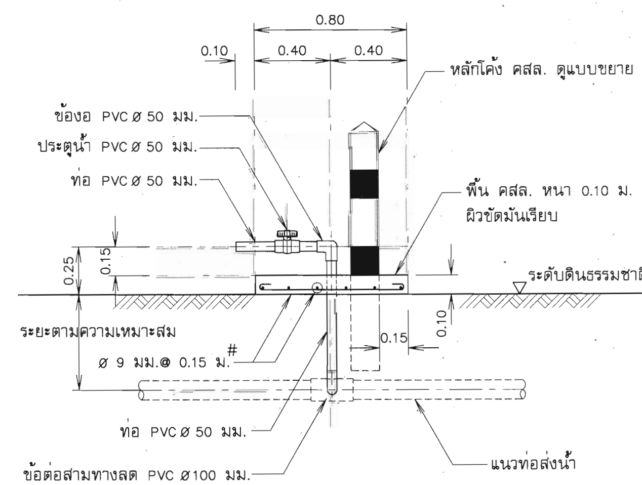
รูปตัด ข - ข แสดงการติดตั้งประตูจุดปล่อยน้ำ
