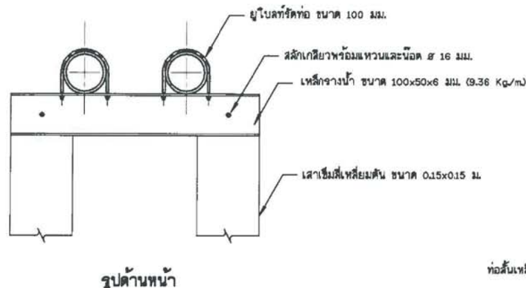
13. เสาค้ำรองรับท่อชุด และแบบขยายอุปกรณ์รัดท่อ ไม่แสดงมาตราส่วน
