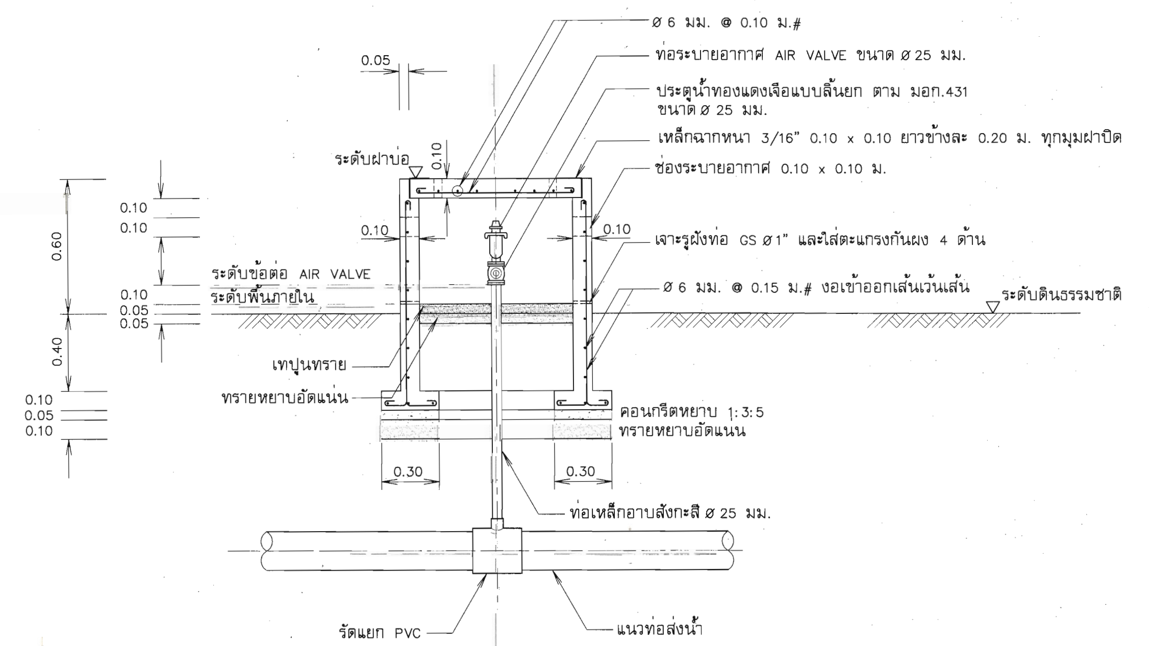
รูปตัด ค - ค แสดงการติดตั้งท่อระบายอากาศ
