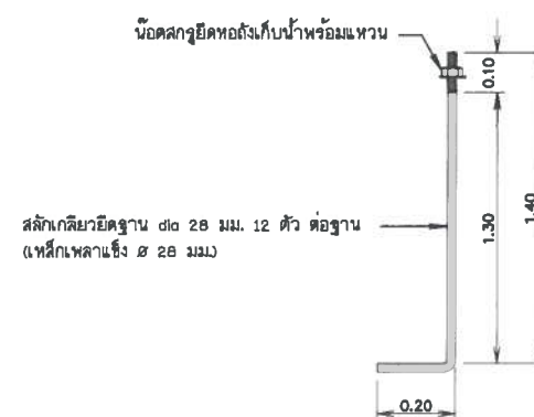
แบบขยายหลักเกลิวยึดฐาน
