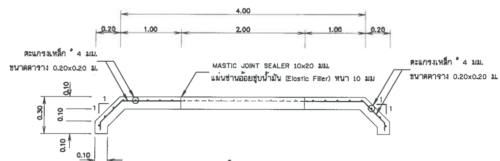
สรุปตัด ค-ค
