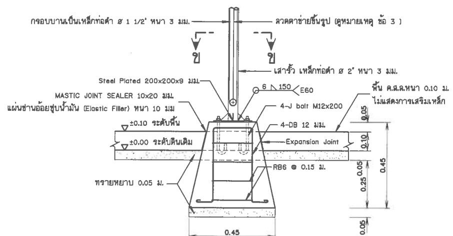
รูปขยายฐานรากโครงสร้างรับแผง F1 (ต่อม่อ คสล. ห่อสำหรับรูปพร้อมติดตั้ง) ไม่แสดงมาตราส่วน
