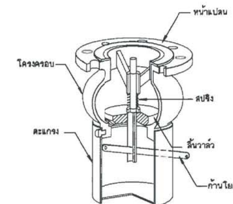
ชุดวาล์ว แบบก้านโยก ไม่แสดงมาตราส่วน
