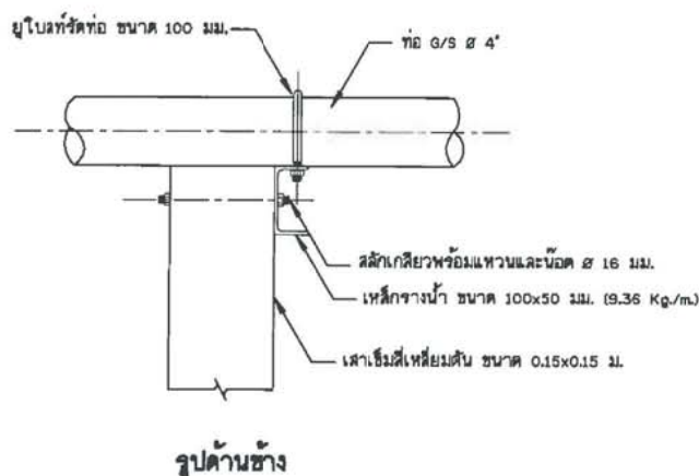
13. เสาคอมมิวนิตี้ท่อชุด และแบบขยายอุปกรณ์รัดท่อ ไม่แสดงมาตราส่วน
