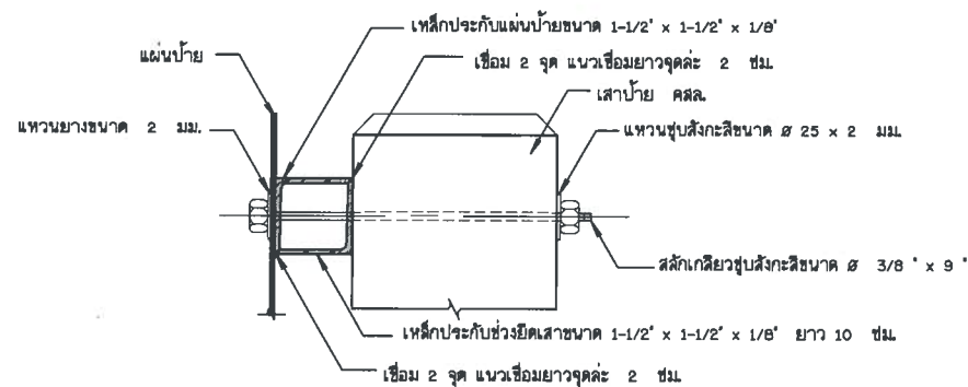
รูปขยายการยึดแผ่นป้ายและเสา ไม่แสดงมาตราส่วน
