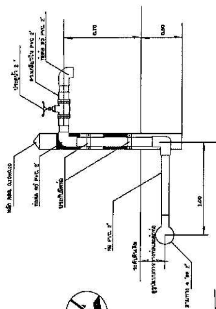
แบบขยายจุดปล่อยน้ำ
