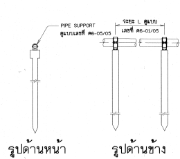
คอมม่อรับท่อแบบที่ 1
