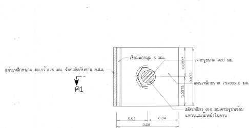
แปลนแผ่นหลักยึดท่อ ไม่แสดงมาตราส่วน
