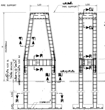
รูปตัดตามขวาง
