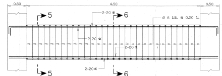
คาน B8 มาตราส่วน 1:25
