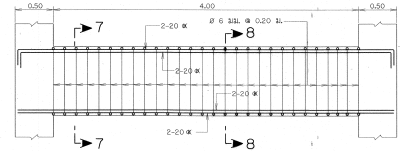
คาน B9 มาตราส่วน 1:25
