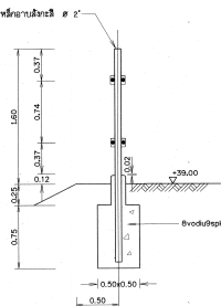
แบบขยายรั้ว (รูปด้านข้าง)
