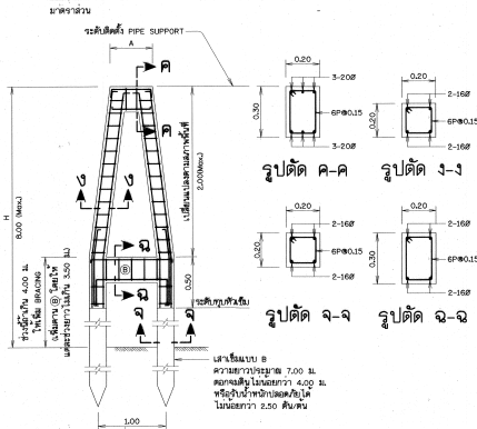
การเสริมเหล็ก คอมม่อแบบที่ 2
