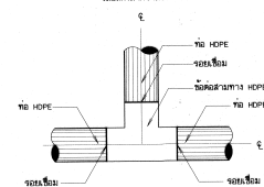
การบรรจบท่อสามทาง HDPE กับท่อ HDPE
