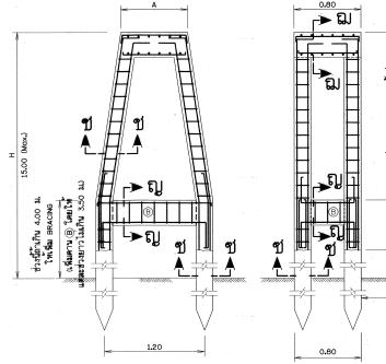
คอมม่อรับท่อแบบที่ 2
