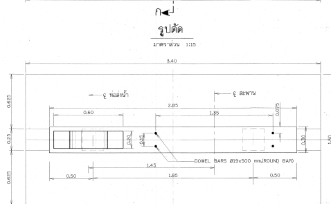
แปลน (รายละเอียดคานด้านล่าง)
