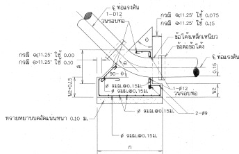
รูปตัด จ-จ
