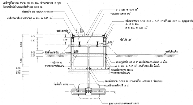
ฉลุตัด ก - ก มาตราส่วน 1:20
