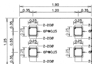
รูปตัด ก-ก
