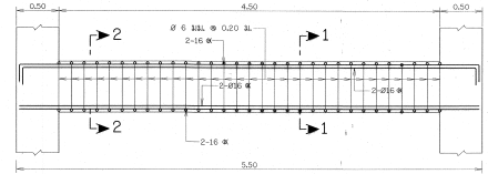
คาน B6 มาตราส่วน 1:25
