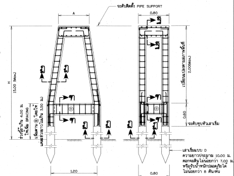
การเสริมเหล็ก คอมม่อแบบที่ 4
