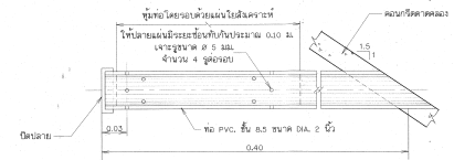
รูปขยาย 3 หรือระบายน้ำ WEEPHOLE ไม่แสดงมาตราส่วน
