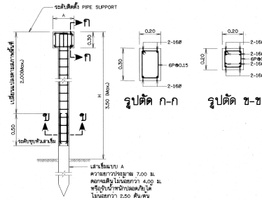
การเสริมเหล็ก คอมม่อแบบที่ 1
