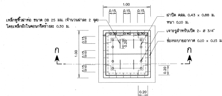
แปลน มาตราส่วน 1:20
