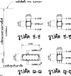
คอมม่อรับท่อแบบที่ 3,4
