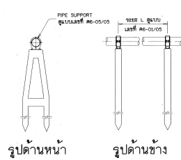
คอมม่อรับท่อแบบที่ 2
