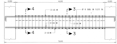
คาน B7 มาตราส่วน 1:25
