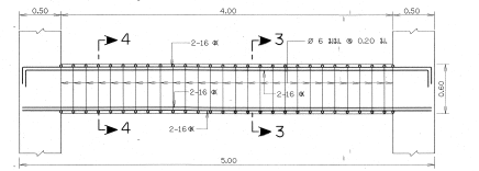
คาน B7 มาตราส่วน 1:125
