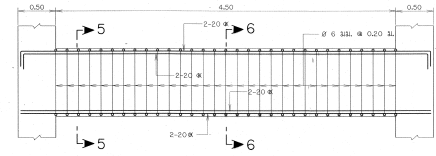
คาน B8 มาตราส่วน 1:125
