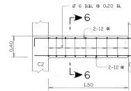
รูปตัด 6-6
