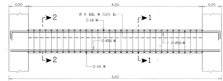
คาน B6 มาตราส่วน 1:125
