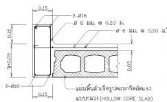
รูปขยาย 4 ไม่แสดงมาตราส่วน
