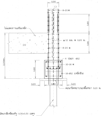
รูปตัดฐานราก, คานคอดิน มาตราส่วน 1:125
