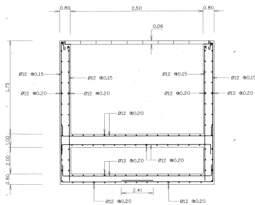
รูปตัด ก-ก มาตราส่วน 1:125
