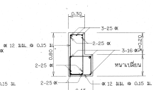
รูปตัด 6-6
