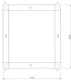
แปลนคานายึด มาตราส่วน 1:150
