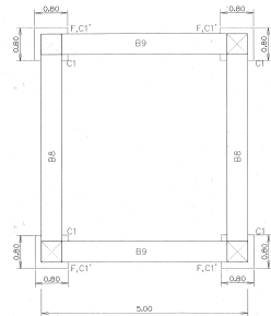
แปลนฐานราก, คานคอดิน มาตราส่วน 1:150
