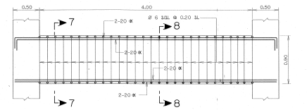
คาน B9 มาตราส่วน 1:125
