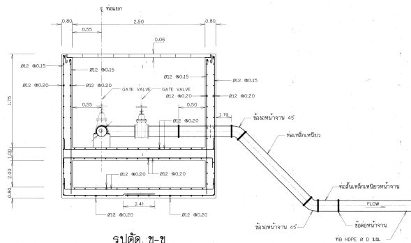
รูปตัด ข-ข มาตราส่วน 1:125
