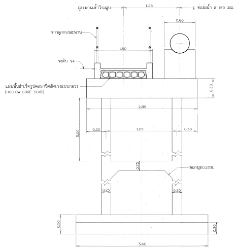
รูปตัด ข - ข มาตราส่วน 1:25
