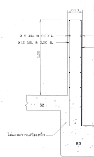
รูปตัด จ - จ
