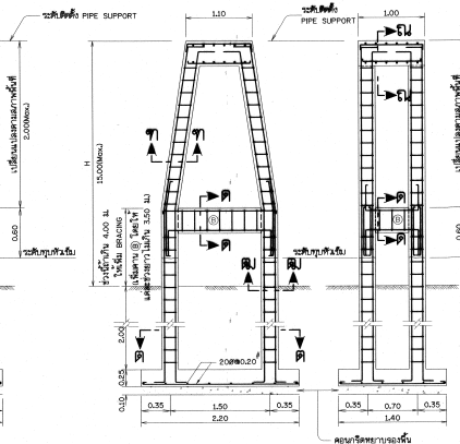
รูปตัดตามขวาง
