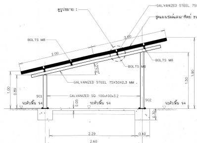
รูปตัด ข - ข
