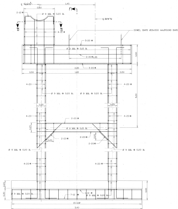
รูปตัด ก มาตรฐาน 1115
