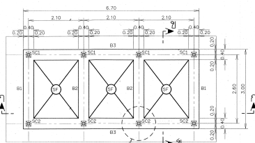
แบบแปลนคานคอดิน
