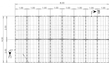
แบบแปลนแผงเซลล์พลังงานแสงอาทิตย์ขนาดไม่น้อยกว่า 310 วัตต์
