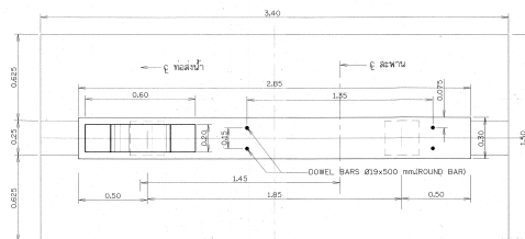
แปลน (รายละเอียดองค์ทาง) มาตรฐาน 1115
