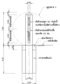
รูปตัด ก-ก แบบที่ 1 แสดง กรมท่อน้ำ ไม่แสดงมาตราส่วน
