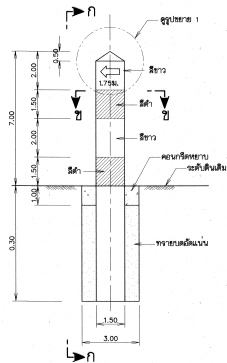
เสา ค.ส.ล. แสดดงแนวทอส่งน้ำ โมเสดมาดจาล้วน
