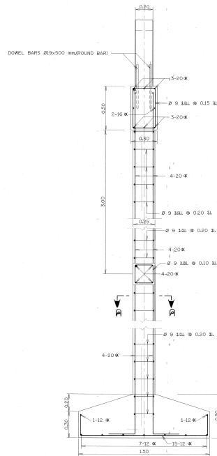
รูปตัด ค - ค มาตรฐาน 1115
