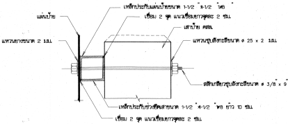
รูปขยายการยึดแผ่นป้ายและเสา มาตราส่วน 1:20
