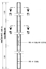
รายละเอียดเสาป้าย คลล มาตราส่วน 1:20
