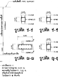
คอมม่อรับท่อแบบที่ 3,4
