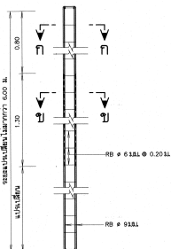
รายละเอียดลำป้าย คลส
