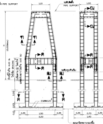
ต่อม่อรับทอแบบที่ 2
