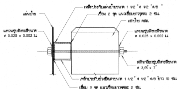
รูปขยายการยึดแผ่นป้ายและลำ
