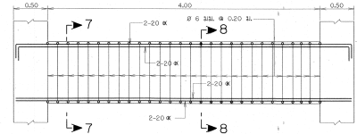
คาน B9 มาตราส่วน 1:25
