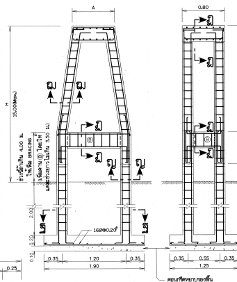
คอม่อรับทอแบบบที่ 1
