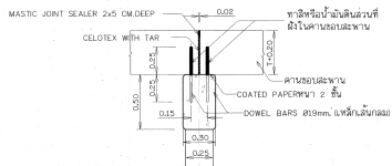
รูปขยาย DOWEL BARS
