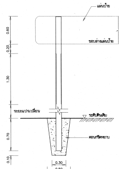
รายละเอียดการติดตั้งลำป้าย
