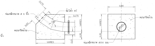
รูปตัด ก1 - ก1 ไม่แสดงมาตรฐาน
