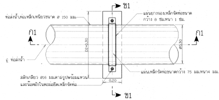
แปลนการยึดท่อ ไม่แสดงมาตรฐาน
