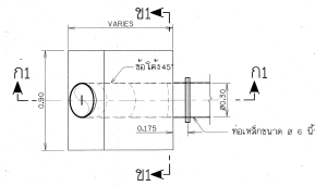
แปลน THRUST BLOCK ไม่แสดงมาตรฐาน
