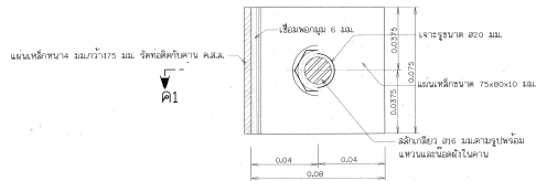
แปลนแผ่นหลักยึดท่อ ไม่แสดงมาตรฐาน
