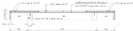
รูปตัดหลังคา คสล. มาตราส่วน 1:120
