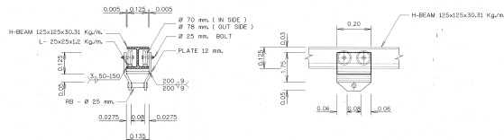
รูปขยาย 1 มาตราส่วน 1:120
