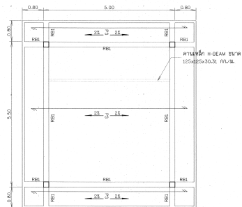
แปลนคาน หลังคา มาตราส่วน 1:250
