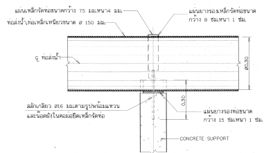
รูปตัด ก1 - ก1 ไม่แสดงมาตรฐาน
