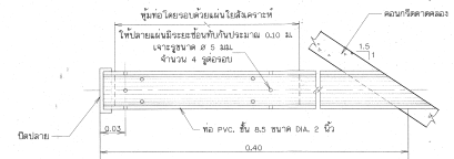
รูปขยาย 3 หรือระบายน้ำ WEEPHOLE ไม่แสดงมาตรฐาน
