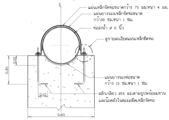
รูปตัด ข1 - ข1 ไม่แสดงมาตรฐาน
