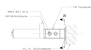
แบบขยาย 1 ขนาดส่วน 1:5
