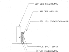
รูปตัด ค - ค ขนาดส่วน 1:5
