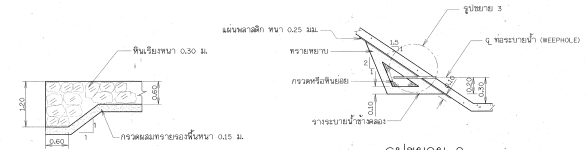
รูปขยาย 1 ไม่แสดงมาตรฐาน
