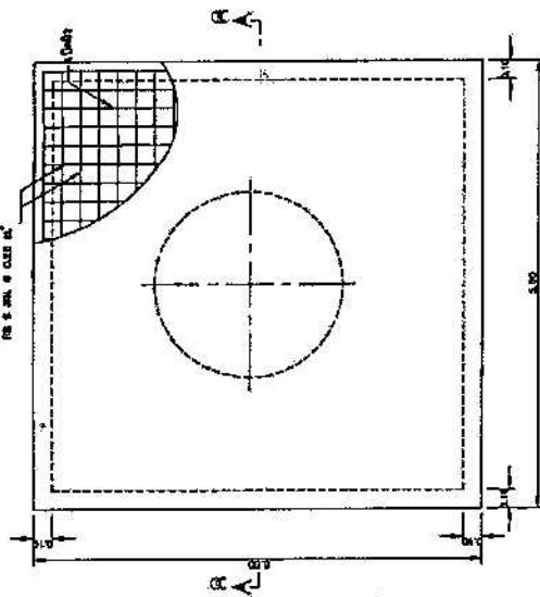
แปลนพิมพ์คอนกรีตเสริมเหล็ก
