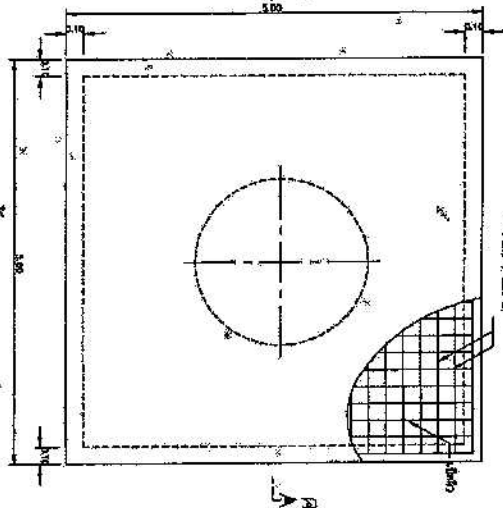
แบบพื้นคอนกรีตเสริมเหล็ก
