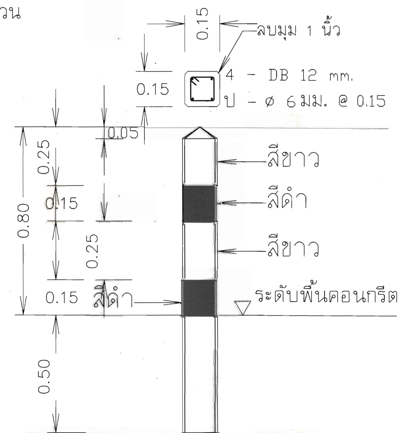
แบบขยายหลักบ่อแนว
