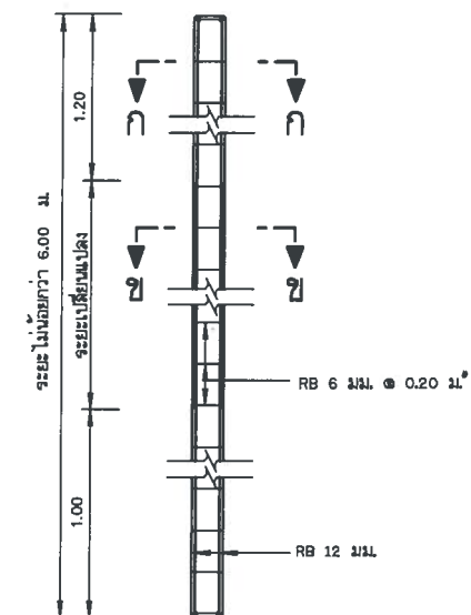
แบบโครงการ ไม่แสดงมาตราส่วน
