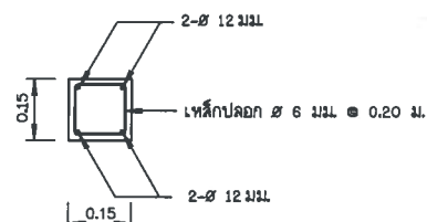
แบบโครงการ ไม่แสดงมาตราส่วน
