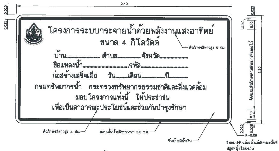
แบบโครงการ ไม่แสดงมาตราส่วน
