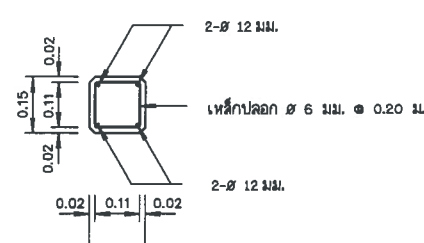
แบบโครงการ ไม่แสดงมาตราส่วน
