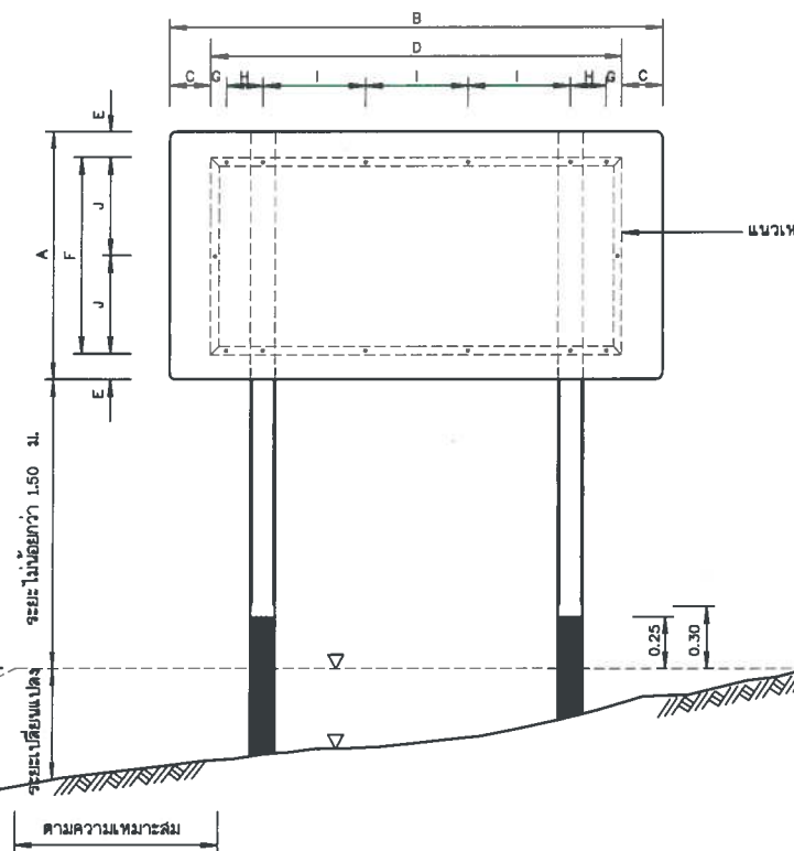
แบบโครงการ ไม่แสดงมาตราส่วน
