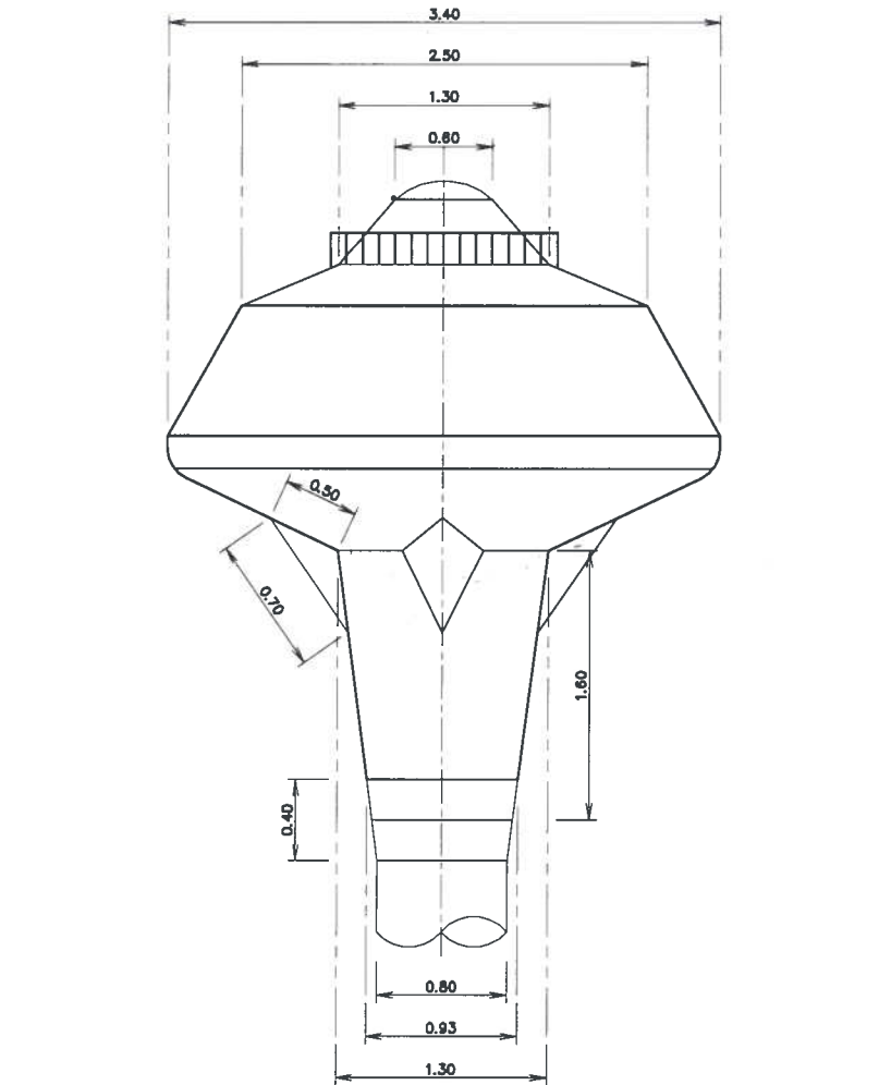
แบบขยายแมนโฮลบนถังสูง ไม่แสดงมาตราส่วน
