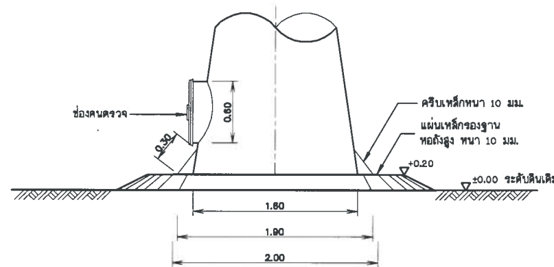
แบบขยายแมนโฮลล่างถังสูง ไม่แสดงมาตราส่วน
