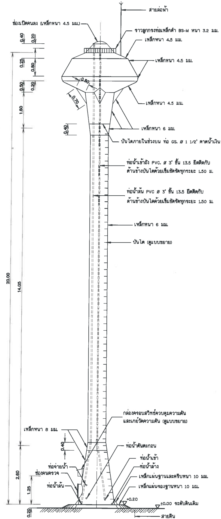
รูปด้านข้างหอดังสูง แบบถึงเหล็กรูปทรงแฉมเปญ
