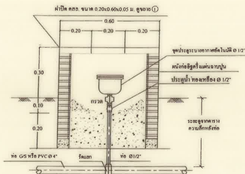
การติดตั้งประตูปะบายอากาศอัตโนมัติ
