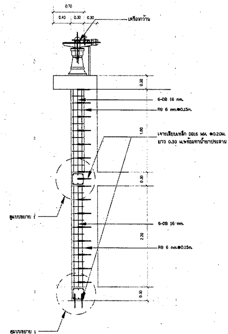
ภาพตัด ข-ข มาตราส่วน 1:50
