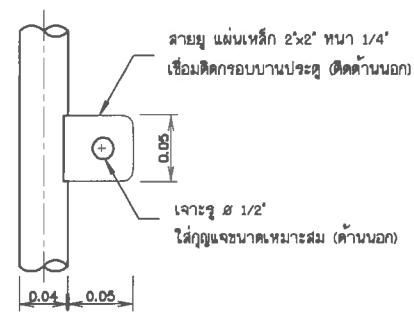
แบบขยายสายยู ไม่แสดงขนาดบางส่วน
