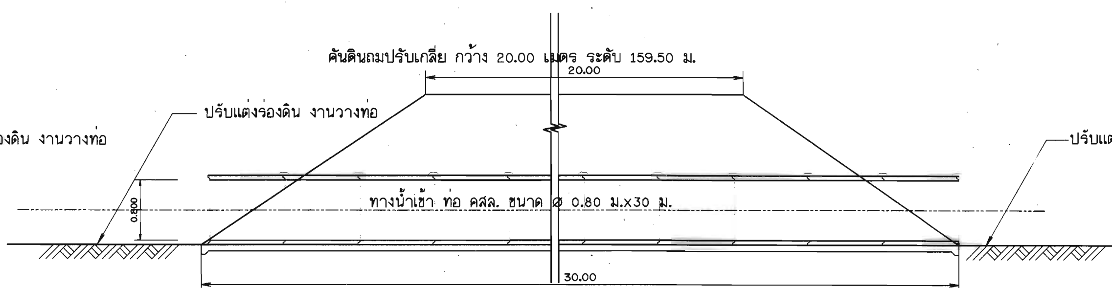
รูปตัด 1 - 1 มาตรฐาน 1:50
