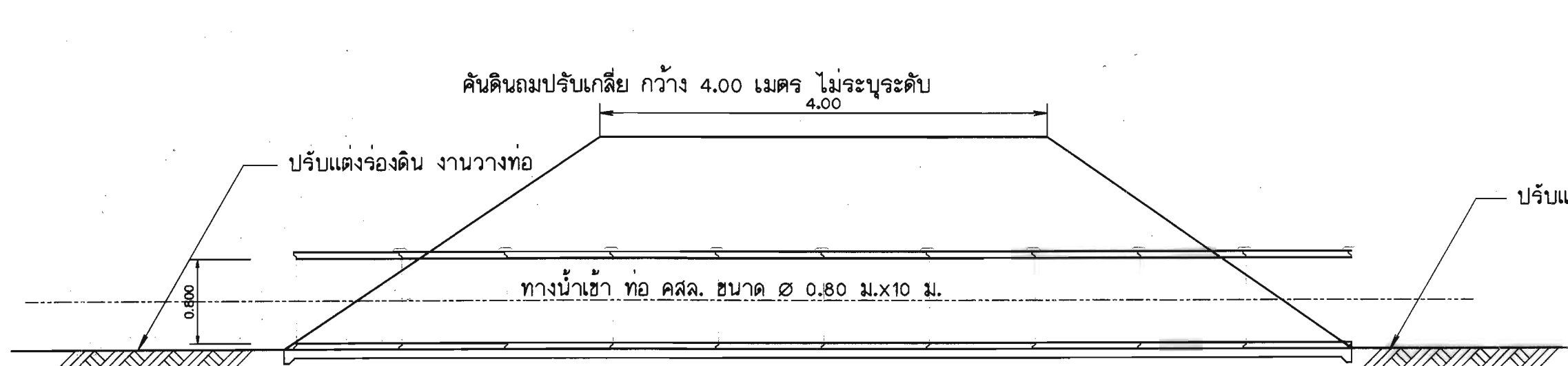
รูปตัด 1 - 1 มาตรฐาน 1:50
