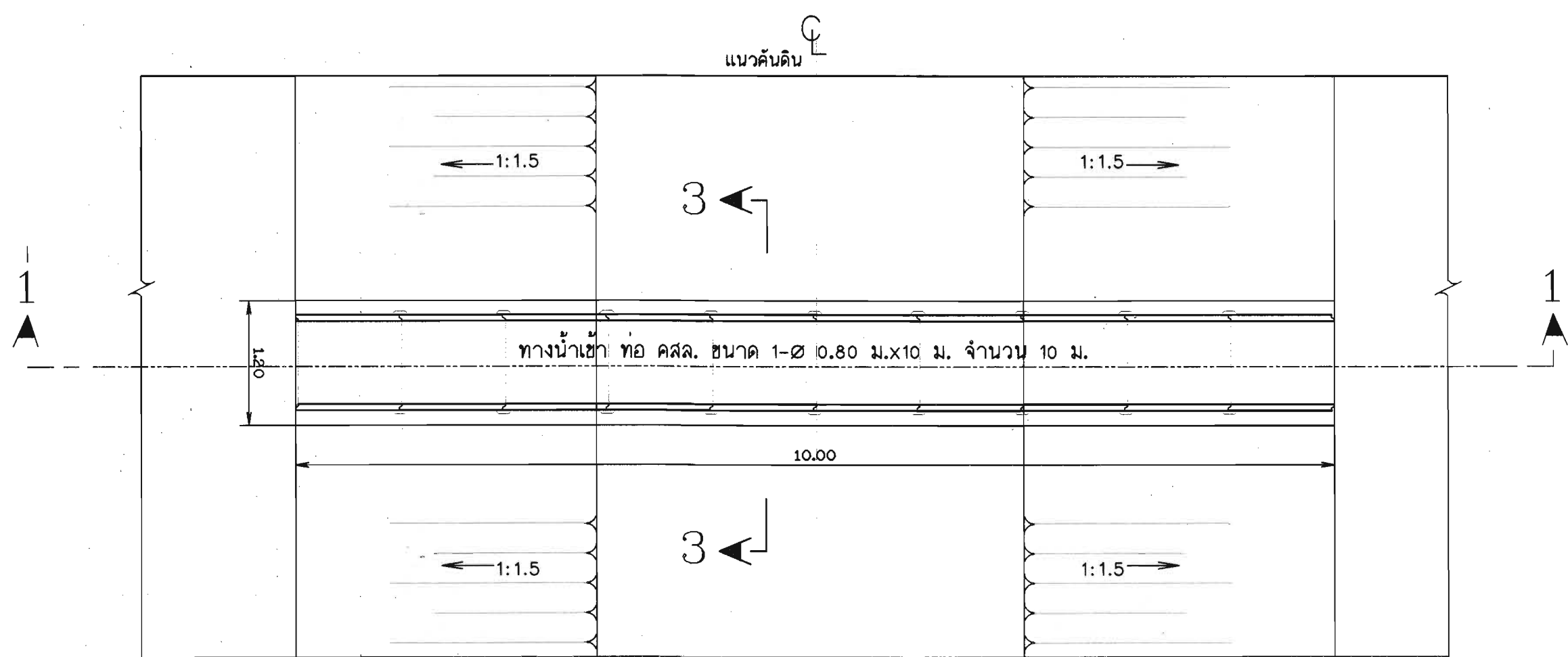
แปลนวางท่อ คสล. ขนาด \varnothing 0.80 ม. (คันดิน กว้าง 4.00 ม.) ③ มาตรฐาน 1:50
