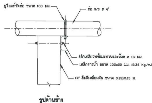
13. เสาค้ำรับท่อวัด และแบบขยายอุปกรณ์รัดท่อ ไม่แสดงมาตราส่วน
