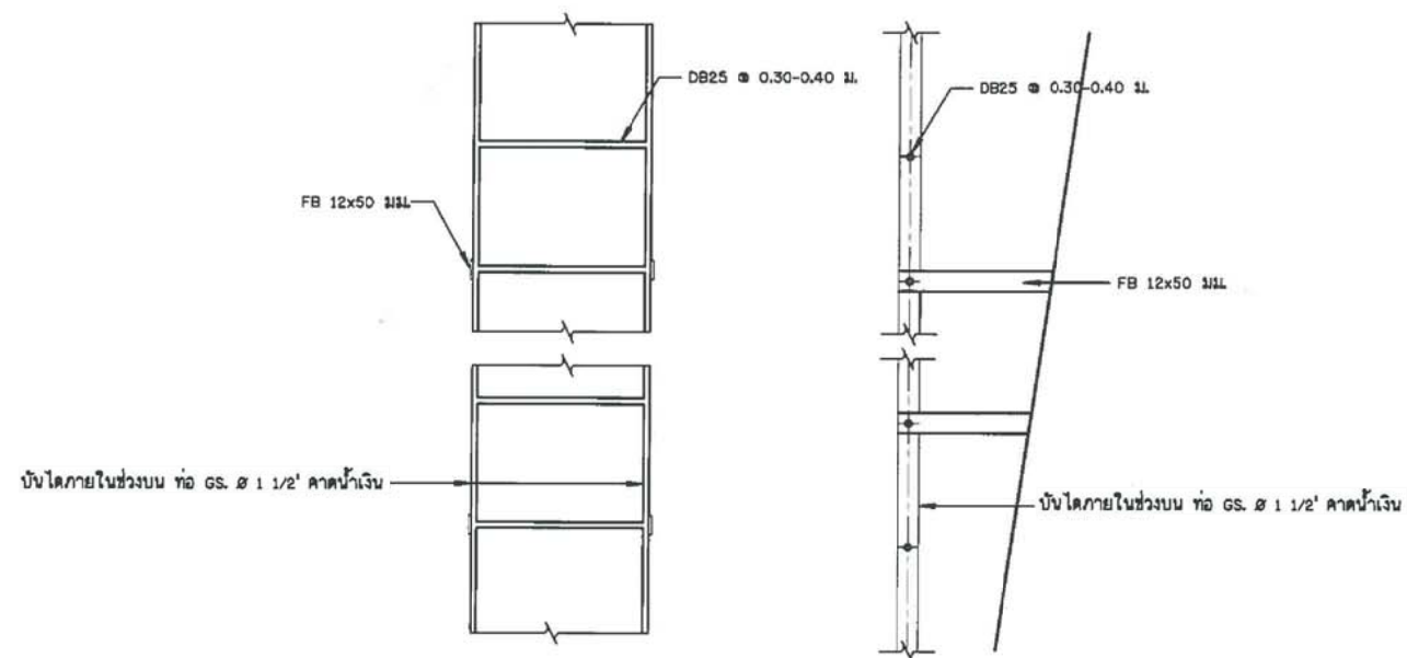
แบบขยายบันได ภายในหอถังสูง ไม่แสดงมาตราส่วน
