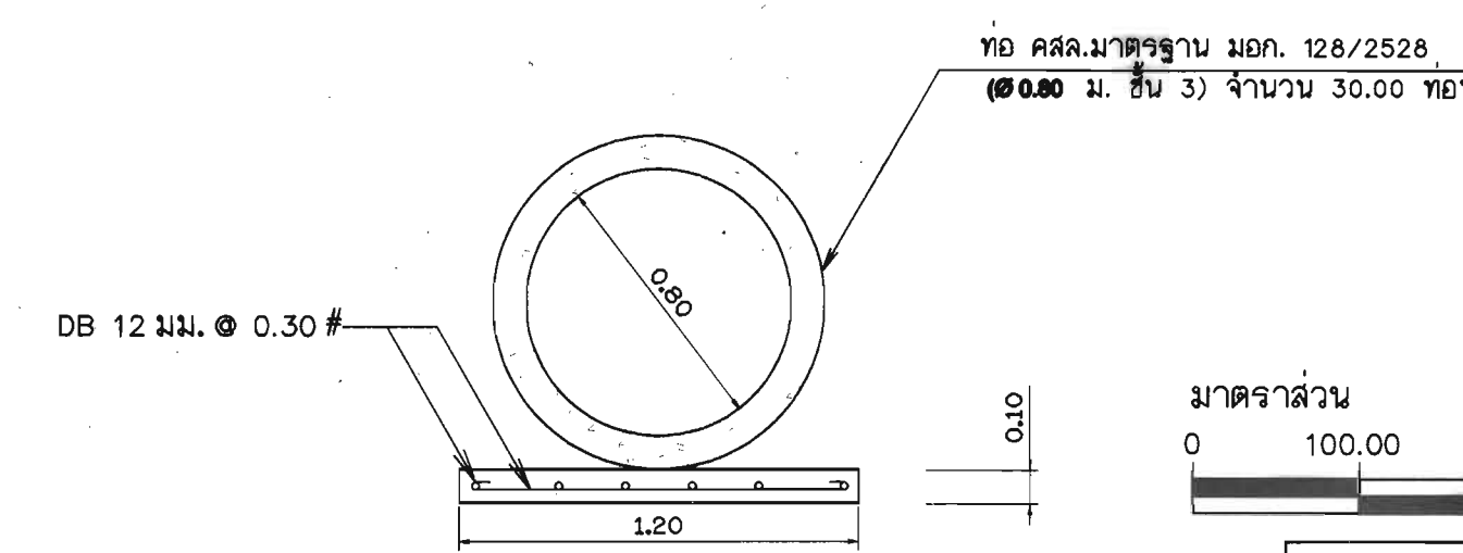
รูปตัด 1 - 1 มาตรฐาน 1:50
