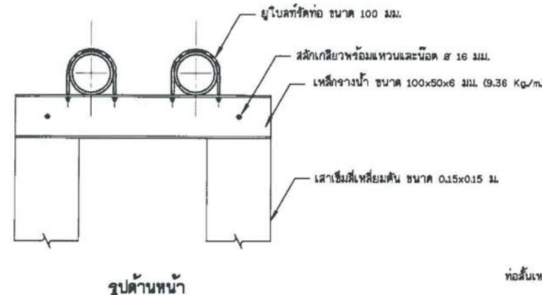
13. เสาค้ำรับท่อวัด และแบบขยายอุปกรณ์รัดท่อ ไม่แสดงมาตราส่วน
