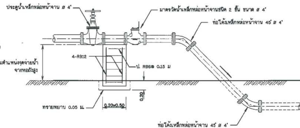
14. การติดตั้งมาตรวัดน้ำบนพื้นดิน 5 4' ไม่แสดงมาตราส่วน
