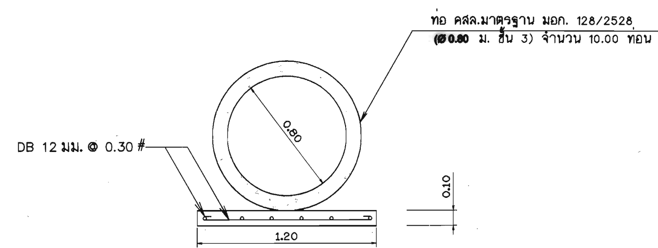
รูปตัด 3 - 3 มาตรฐาน 1:25
