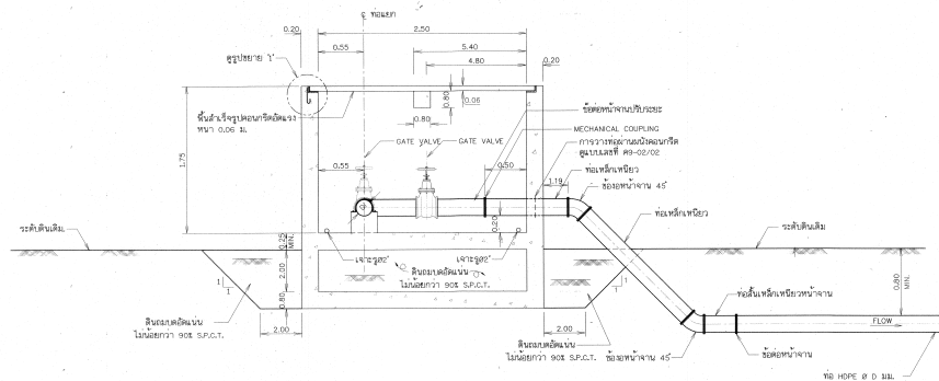
รูปตัด ข-ข
