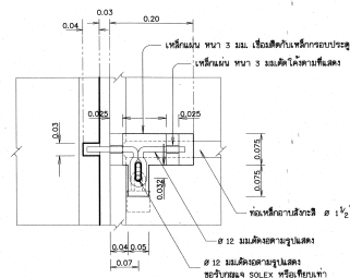
แบบขยายจั่ว 1
