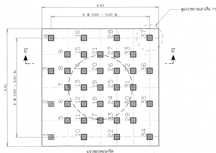
แบบแปลนตำแหน่งเส้นเสริม
