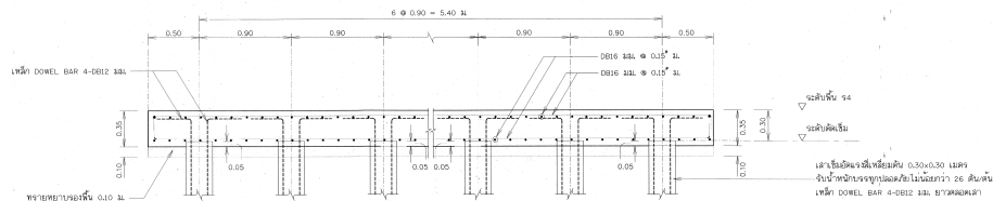
รูปตัด ก1 - ก1
