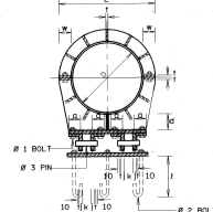
รูปตัด ค-ค
