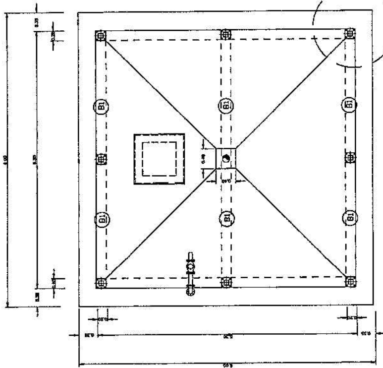
แบบขยายคาน B1
