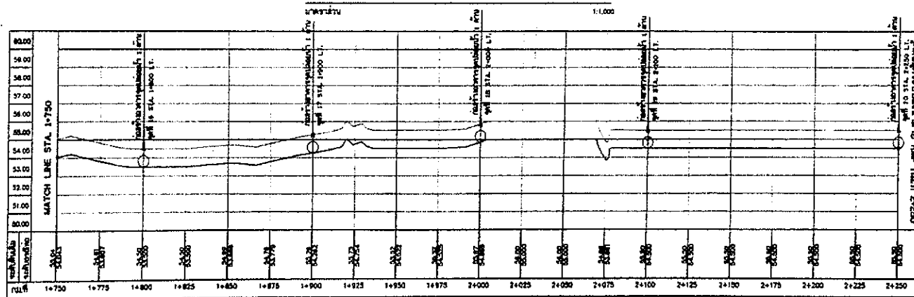
รูปตัดตามยาวระบบส่งน้ำสาย RMP STA.1+750-2+250
