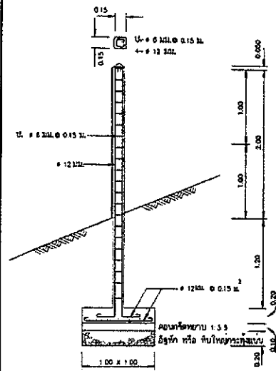
ขยายหน้าตัด ค.ค. ค้ำยันน้ำ
