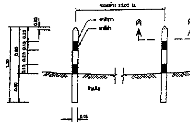
รูปขยายหน้าตัดค้ำยันน้ำ ขนาดหน้าตัด 1:20
