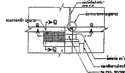
แปลนอาคารบังคับน้ำ
