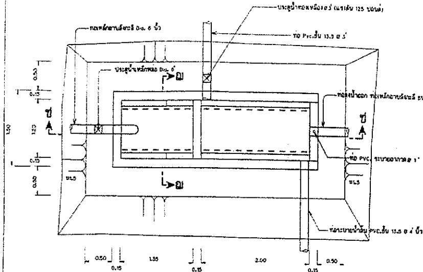
แบบแปลนบ่อตกตะกอน
