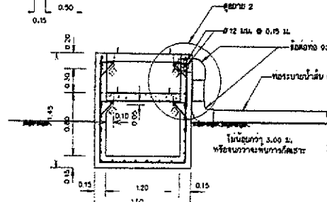
รูปตัด ฉ - ฉ
