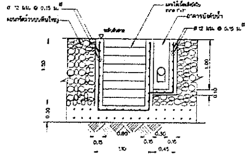
รูปตัด ง - ง
