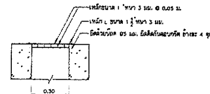
รูปตัด จ - จ
