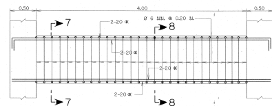
คาน B9 มาตราส่วน 1:25
