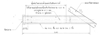
รูปขยาย 3 ท่อระบายน้ำ WEAPHOLE ไม่แสดงมาตราส่วน
