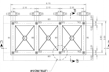
แปลนคานคอดิน
