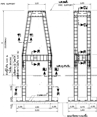
รูปตัดตามขวาง
