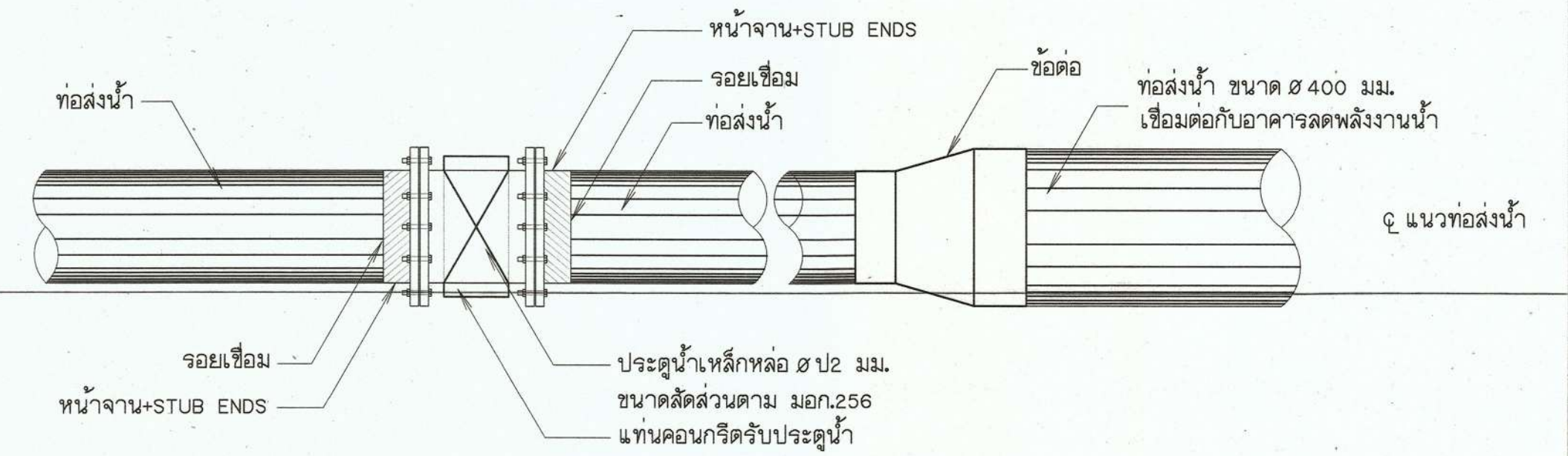
รูปขยายการติดตั้งอาคารควบคุมพลังงานน้ำ มาตราส่วน 1:20
