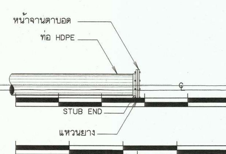
การปิดปลายท่อ
