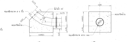
รูปตัด ก1 - ก1 ไม่แสดงมาตราส่วน
