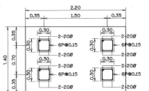
รูปตัด ต-ต
