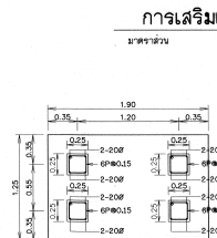
รูปตัด ข-ข
