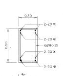
รูปตัด 12-12 มาตราส่วน 1:25
