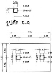
รูปตัดตามขวาง
