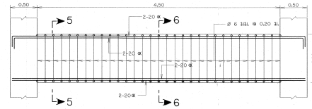
รูปตัด 7-7 มาตราส่วน 1:25
