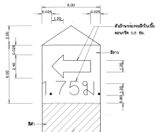
รูปขยาย 1 ไม่ว่าขนาดถ้วน
