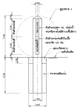
รูปตัด ก-ก แบบที่ 1 แสดง กว.ที่ส่งน้ำ ไม่แสดงขนาดราวน
