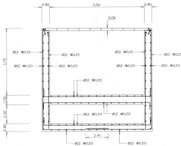
รูปตัด ก-ก มาตรฐาน 1:25
