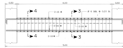
คาน B7 มาตราส่วน 1:25
