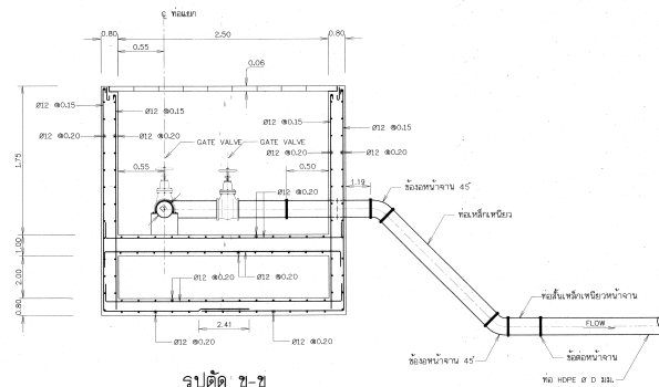
รูปตัด ข-ข มาตรฐาน 1:25
