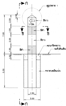
เสา ค.ส.ล. แสดงแนวท่อส่งน้ำ โมเดลมาตราส่วน
