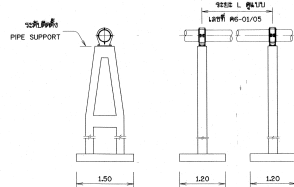
รูปด้านหน้า
