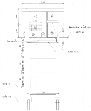
รูปด้าน (1) มาตรฐาน 1:75
