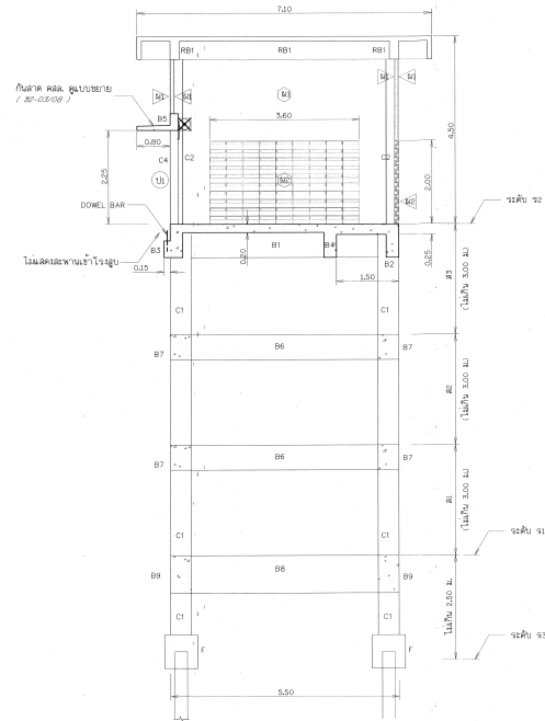
รูปตัด ก - ก มาตรฐาน 1:50
