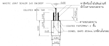
รูปขยาย DOWEL BARS ไม่ลดมาตราส่วน
