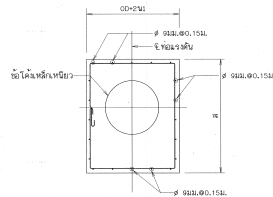
รูปตัด ช-ช
