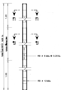
รายละเอียดส่าย คสล.
