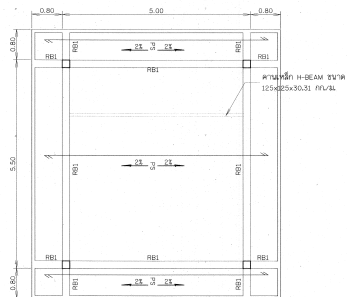
แปลนคาน พื้นหลังคาน
