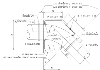
รูปตัด ฉ-ฉ
