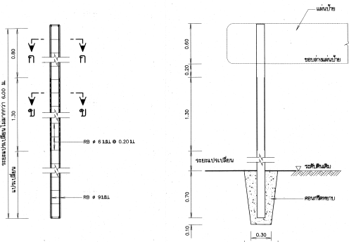
รายละเอียดเสาป้าย คลส
