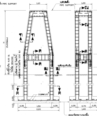
รูปตัดตามขวาง
