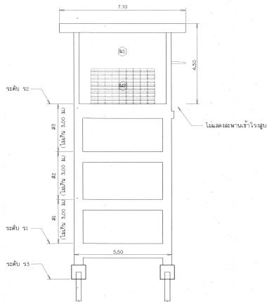
รูปด้าน (2) มาตรฐาน 1:75
