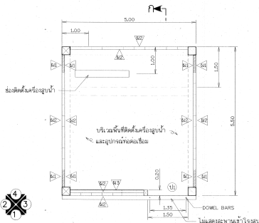
แปลนพื้น
