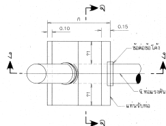
แบบฉนวน
