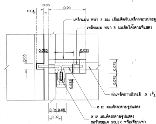
แบบขยาย 1
