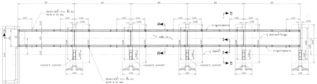
แปลน มาตราส่วน 1:50
