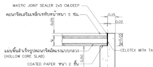
รูปขยาย 3 ไม่ลดมาตราส่วน
