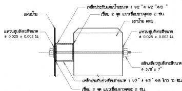
รูปขยายการขีดเส้นแถมป้ายและเสา
