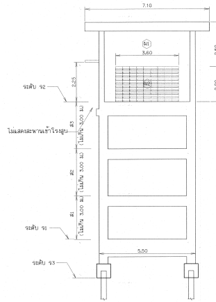
รูปด้าน (3) มาตรฐาน 1:75
