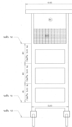
รูปด้าน (4) มาตรฐาน 1:75
