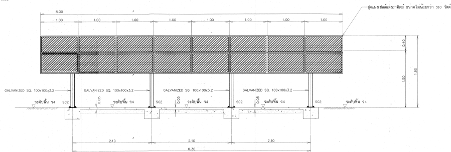
รูปตัด ก - ก
