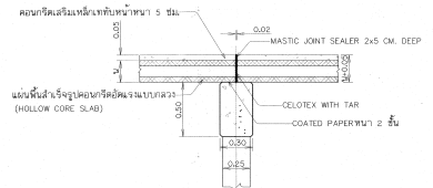
รูปขยาย 2 ไม่ลดมาตราส่วน
