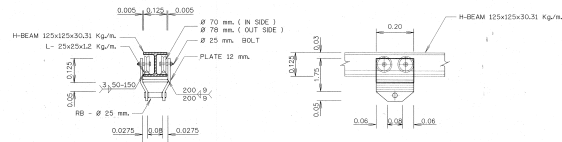
รูปขยาย 1
