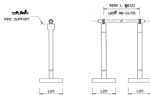
รูปตัดหน้า
