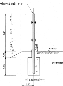
แบบขยายรั้ว (รูปด้านข้าง)
