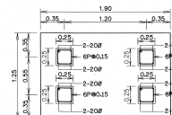
รูปตัด ข-ข
