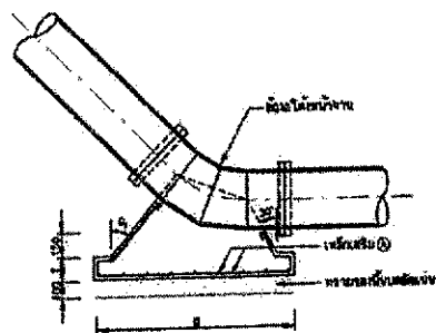
รูปตัด ข-ข
