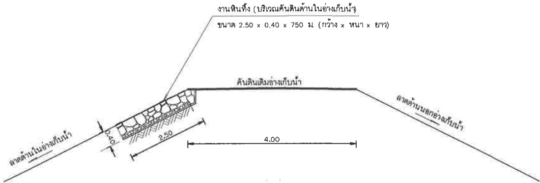
รูปตัด ก - ก
