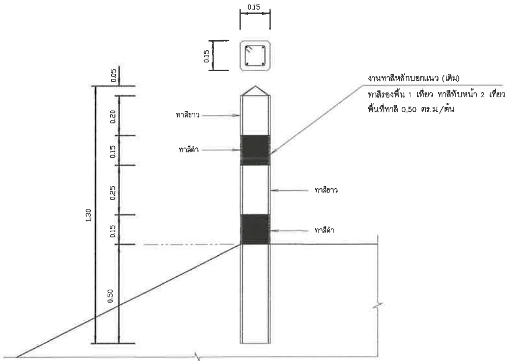
แบบขยายหลักบอแก้ว (งานทาสีหลักบอแก้วเดิม)
