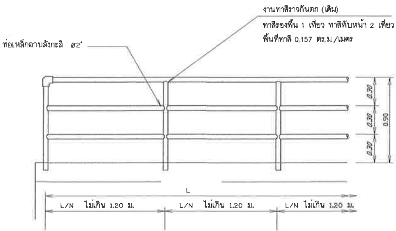
รูปขยายเหล็กขาวกันตก (งานทาสีขาวกันตกเดิม)
