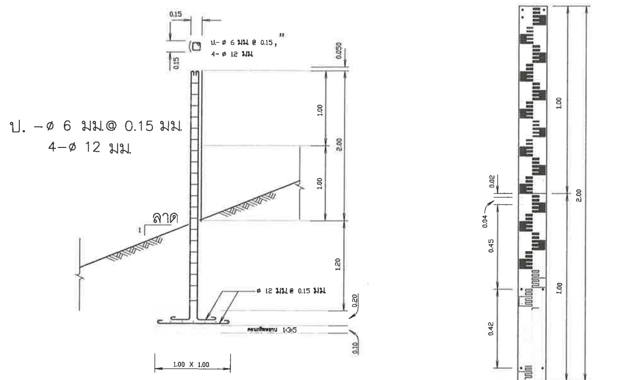
ขยายหลัก คสล. บอกค่าระดับ
