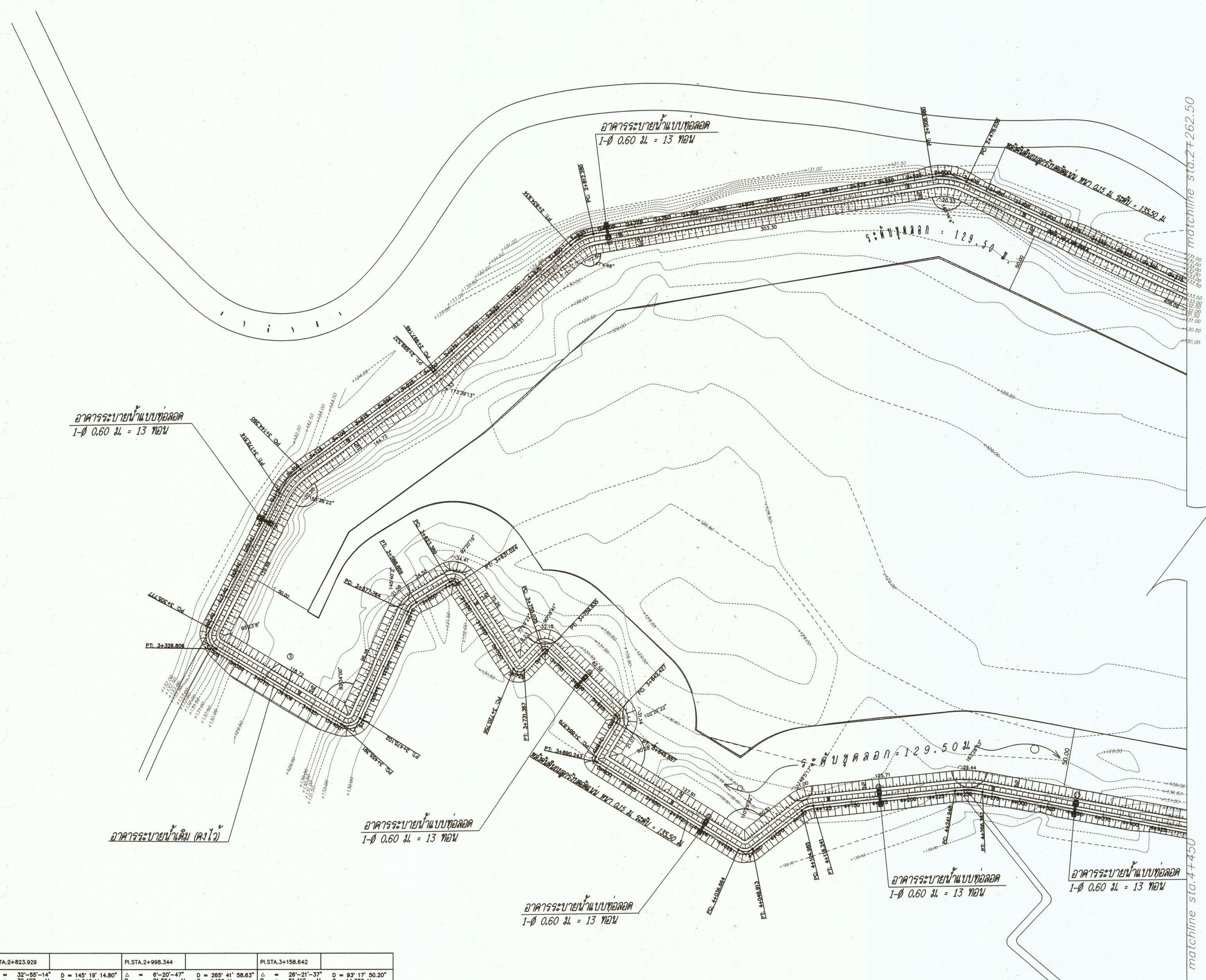
General plan มาตราส่วน 1:2,000
