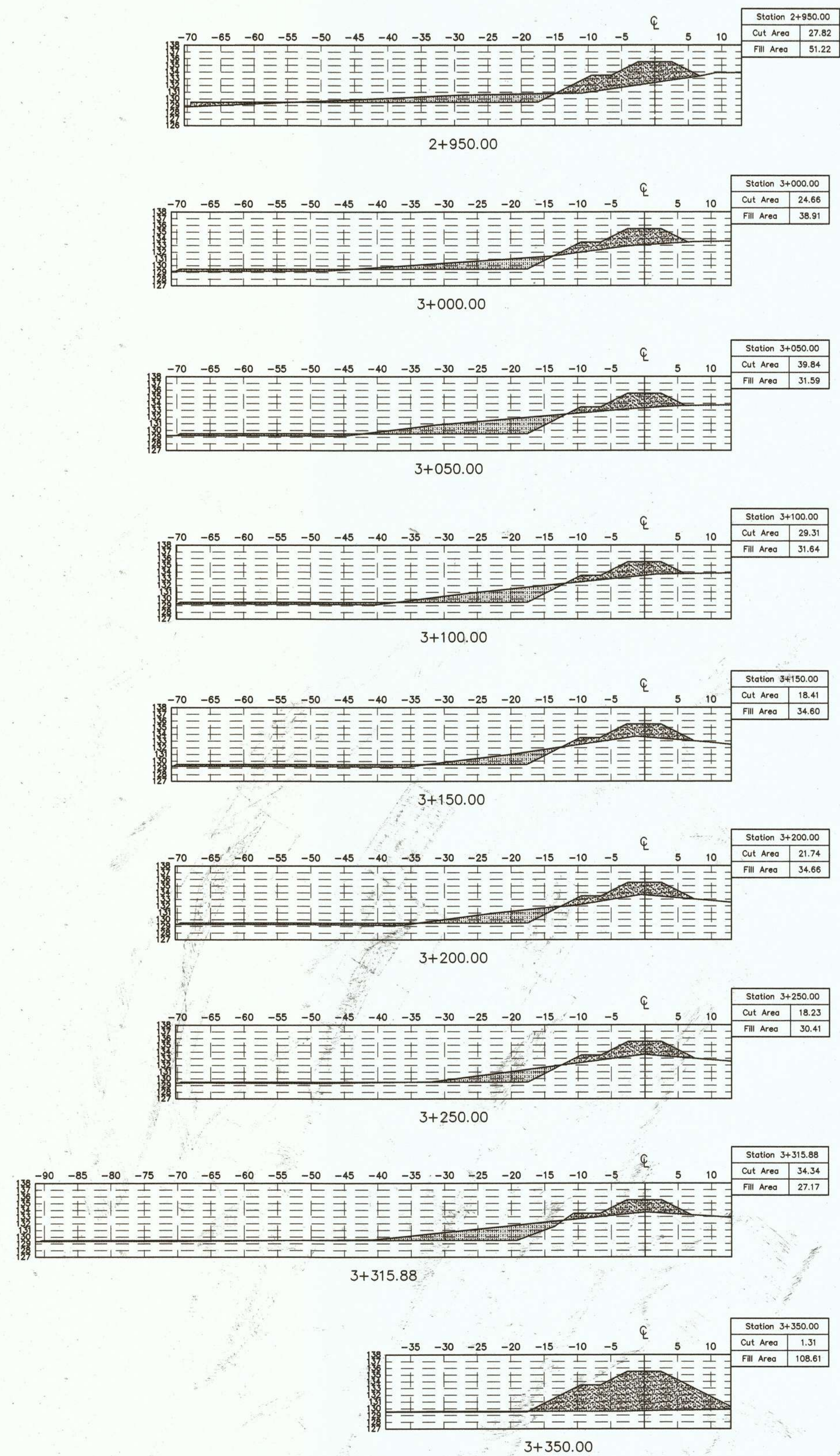
Cross Section มาตราส่วน 1:500
