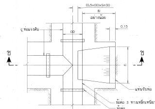
แปลน
