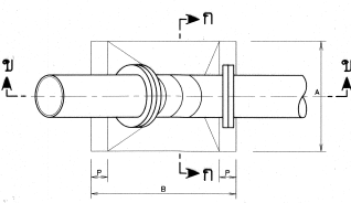
แปลน THRUST BLOCK รับข้อต่อโค้งแนวตั้ง
