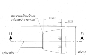
แปลน
