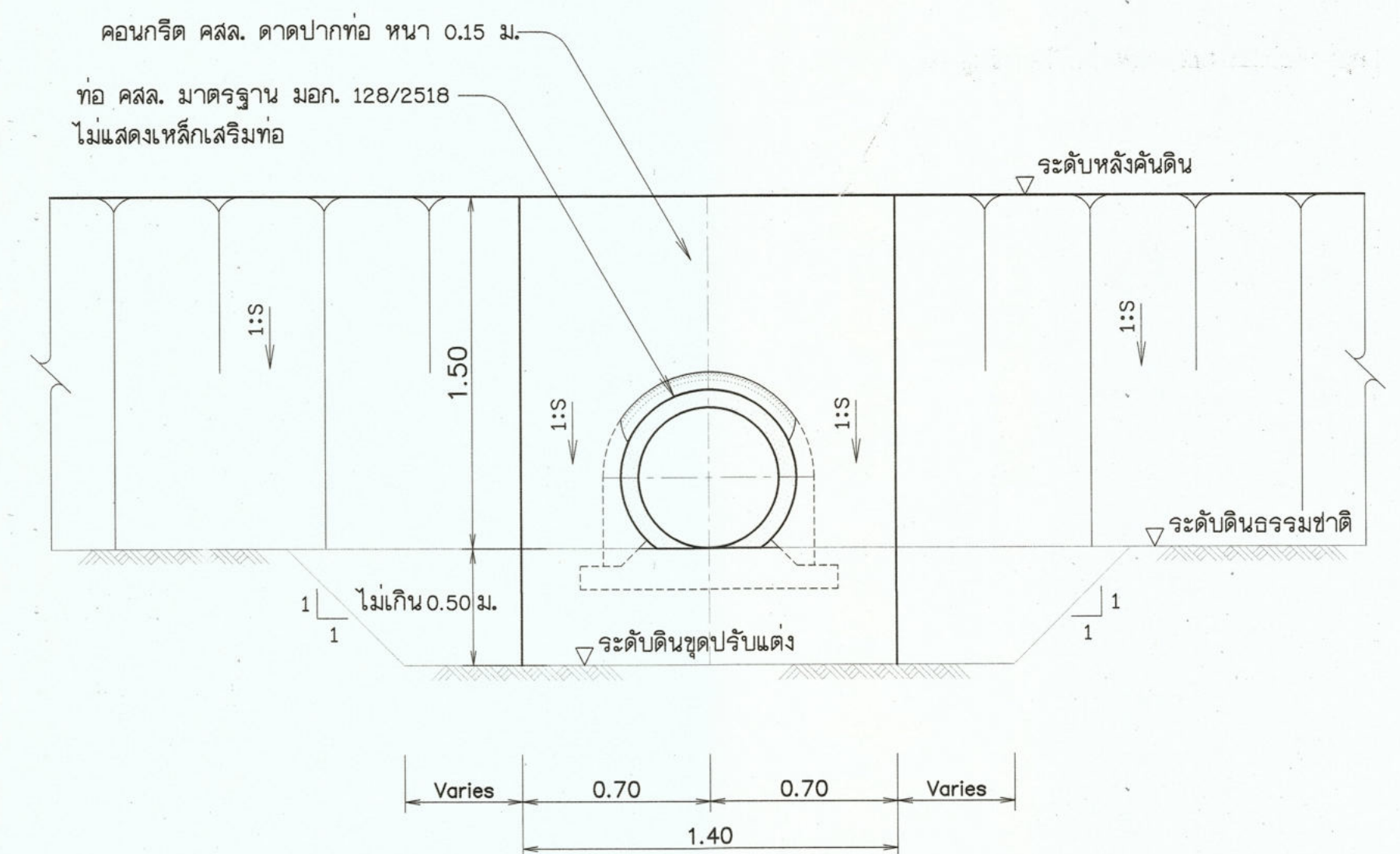
แบบปากทางน้ำเข้าอาคารทอลอดคั่นดิน
