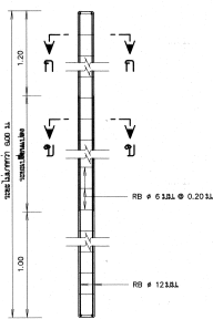
รายละเอียดเสาป้าย คลล.
