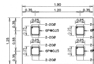
รูปตัด ก-ก
