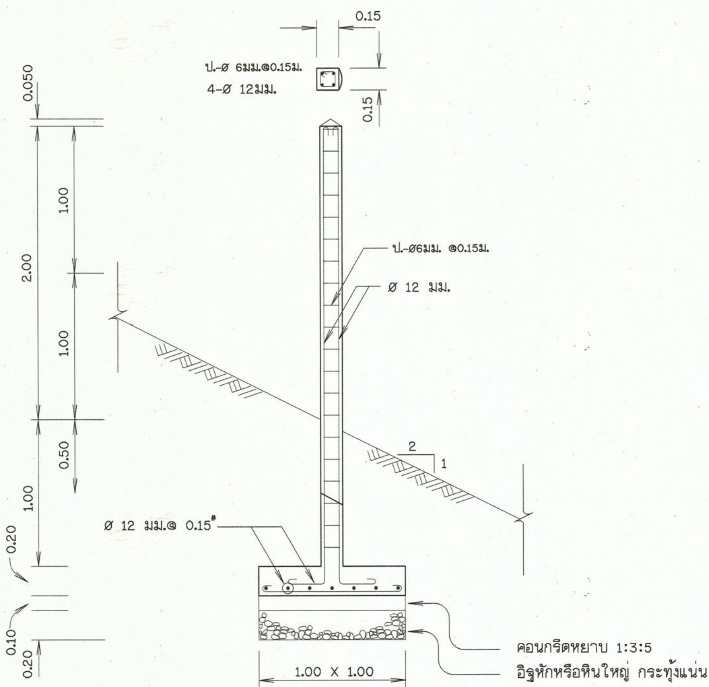
ขยายหลัก คสล.บอกค่าระดับ
