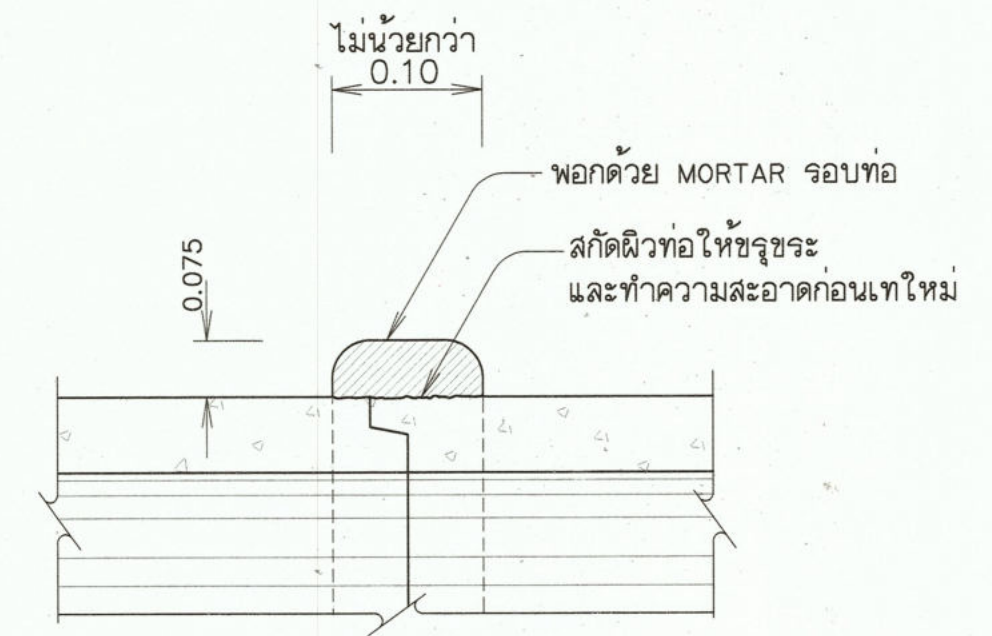
ขยาย ①
