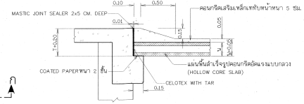
รูปขยาย 1 ไม่ลดมาตราส่วน
