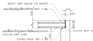
รูปขยาย 3 ไม่ลดมาตราส่วน
