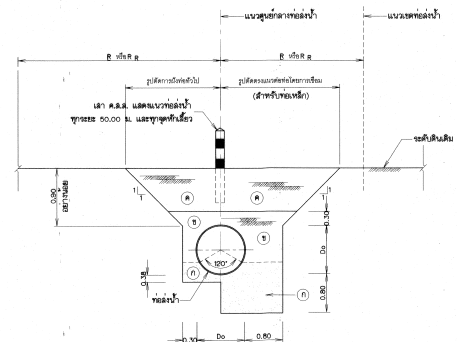
รูปตัดขวางการฝังท่อเหล็กเส้นยว (SP)
