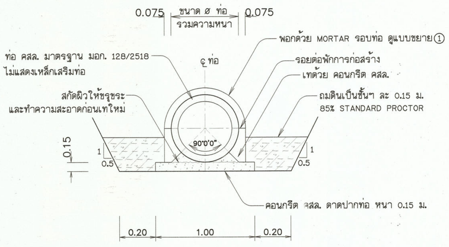
รูปตัดแนว ข - ข
