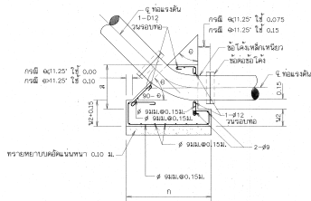
รูปตัด จ-ง มาตราส่วน 1:10
