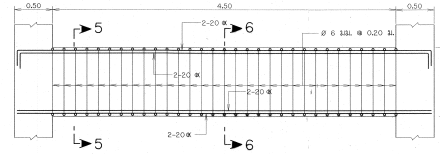
คาน B8 มาตราส่วน 1:25
