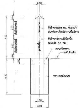
รูปตัด ก-ก แบบที่ 2 แสดงจุดหักเห ไม่แสดงมาตราส่วน
