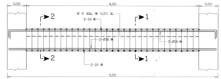
คาน B6 มาตราส่วน 1:25
