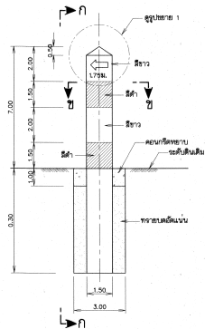
เส้า ค.ส.ล. แสดงแนวท่อน้ำ ไม้แสดงมาดราส่วน
