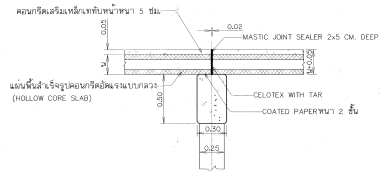
รูปขยาย 2 ไม่ลดมาตราส่วน
