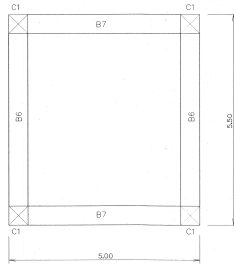
แปลนคานยัด มาตราส่วน 1:150
