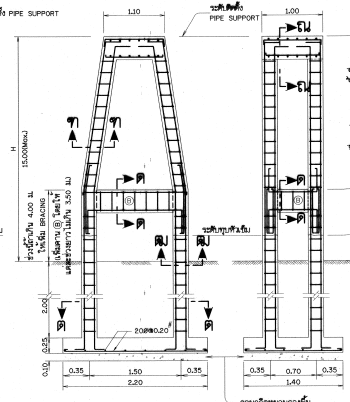
รูปตัดตามขวาง
