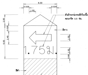
รูปขยาย 1 ไม้มะหาดราลัน
