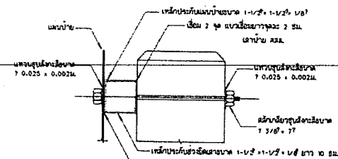
รูปตัดขยายการยึดแผ่นป้ายและเสา ขนาดตัว ๓๒๐
