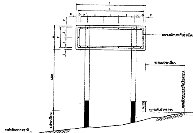
รูปแสดงการประกอบแผ่นป้าย ขนาดตัว ๓๒๐
