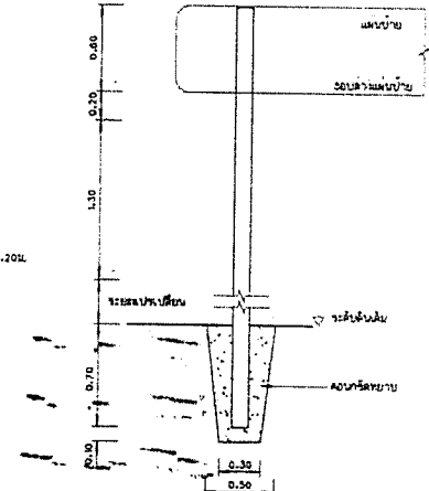
รายละเอียดการติดตั้งเสาป้าย ขนาดตัว ๓๒๐
