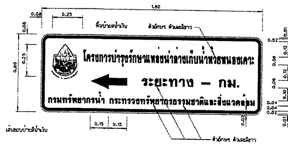
ป้ายแนะนำโครงการ ขนาดตัว ๓๒
