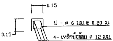
แบบขยายเสา C2 1 : 20
