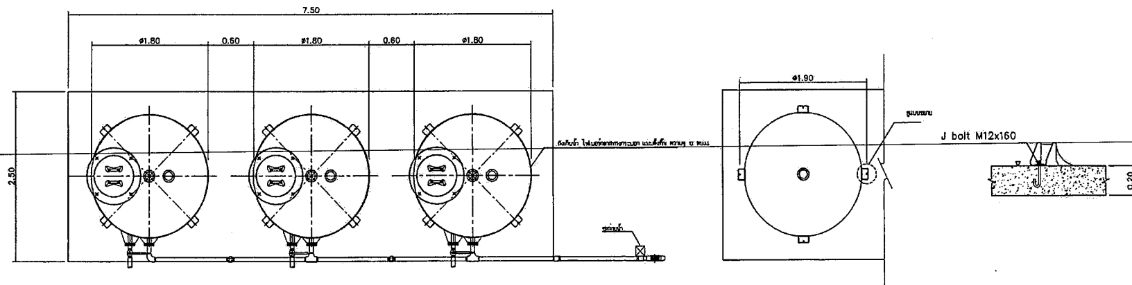
แบบยึดฐาน SCALE: 1:100
