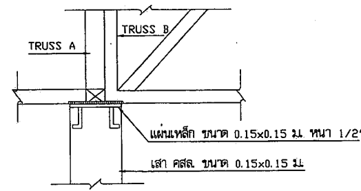
แบบขยายการติดตั้ง TRUSS กับเสา 1 : 10
