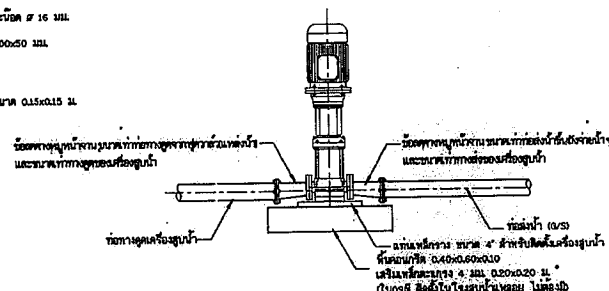
15. การต่อท่อเครื่องสูบน้ำ
