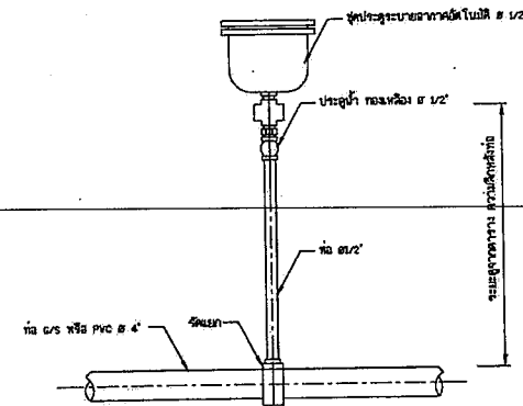
12. การติดตั้งประตูประบายอากาศอัตโนมัติ โมดูลมาตรฐาน
