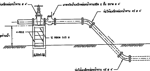
14. การติดตั้งมาตรวัดน้ำบนพื้นดิน ๕' 4" โมดูลมาตรฐาน
