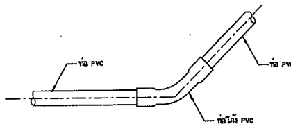
5. แบบการต่อข้อโค้ง 22 1/2, 45° PVC ไม่แสดงมาตรฐาน
