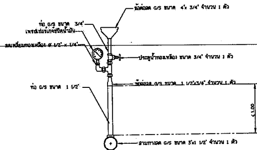
11. ข้องเติมน้ำ โมดูลมาตรฐาน
