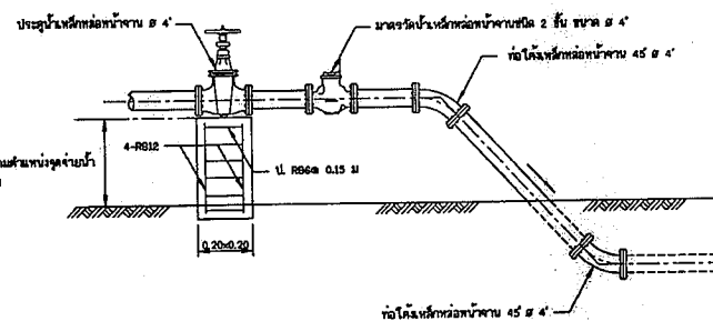
14. การติดตั้งมาตรวัดน้ำบนพื้นดิน ๕ 4"
