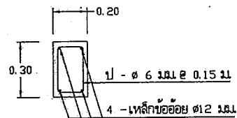
แบบขยายคาน GB 1 : 20
