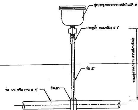
12. การติดตั้งประตูระบายอากาศอัตโนมัติ
