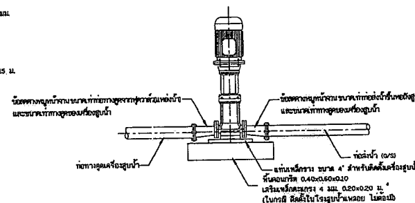
15. การต่อท่อเครื่องสูบน้ำ โมดูลมาตรฐาน
