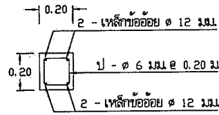
แบบขยายเสา C1 1 : 20
