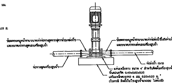
15. การต่อท่อเครื่องสูบน้ำ ไม่ลดขนาดหัว
