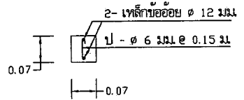
แบบขยายเสา C3 1 : 10
