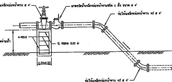
14. การติดตั้งมาตรวัดน้ำบนพื้นดิน ๒ ๔" ไม่ลดขนาดหัว
