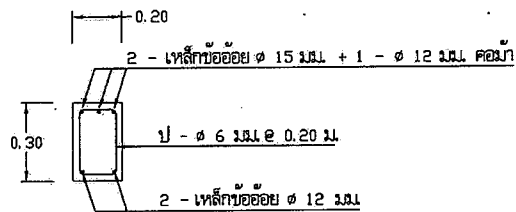
แบบขยายคาน B1 1 : 20
