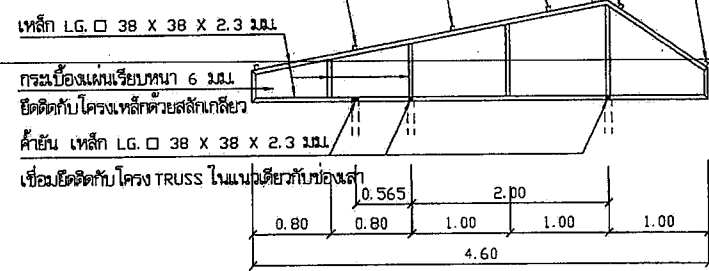
แบบขยาย โครงเหล็กคานข้าง 1 : 50
