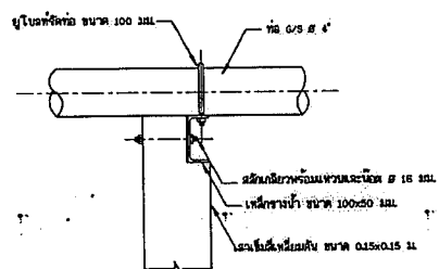
รูปด้านข้าง
