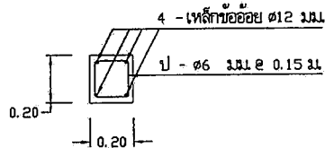
แบบขยายคาน B1 1 : 20
