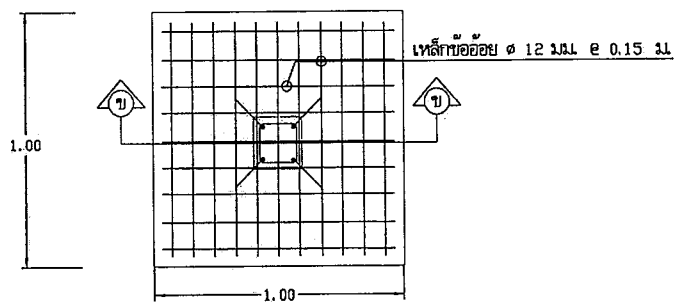
แบบขยายฐานราก F 1 : 20
