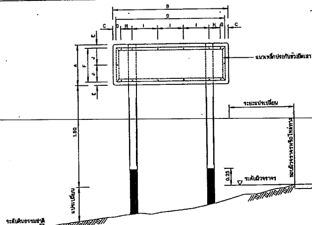
รูปแสดงการประกอบแผ่นป้าย ไม่แสดงมาตราส่วน
