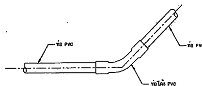
5. แบบการต่อข้อโค้ง 22 1/2, 45° PVC ใบเสนอราคาส่วน
