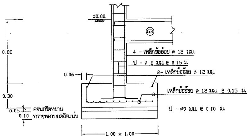
แบบขยายเสา C1 1 : 20
