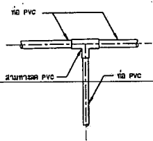
9. แบบการต่อสามทางลด PVC โมดูลมาตรฐาน
