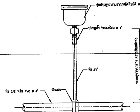
12. การติดตั้งประตูปะบายอากาศอัตโนมัติ ไม่ลดขนาดหัว
