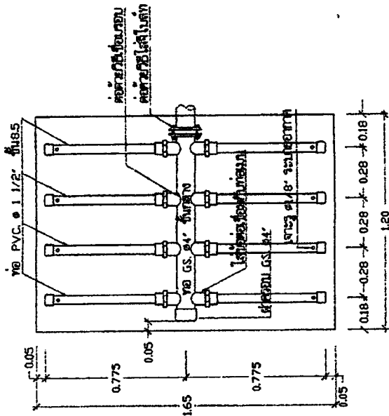
แบบขยายท่อทางปลา 1:20
