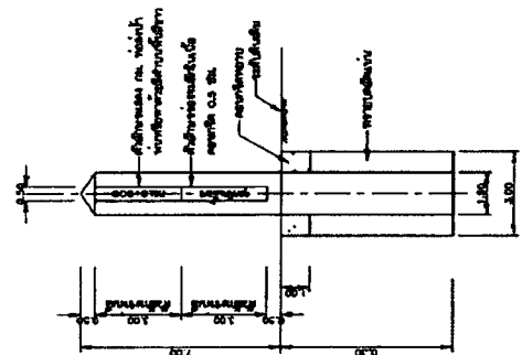
รูปตัด ก-ก แบบ 2 ของชุดสินค้า ไปรษณีย์ ๖๗
